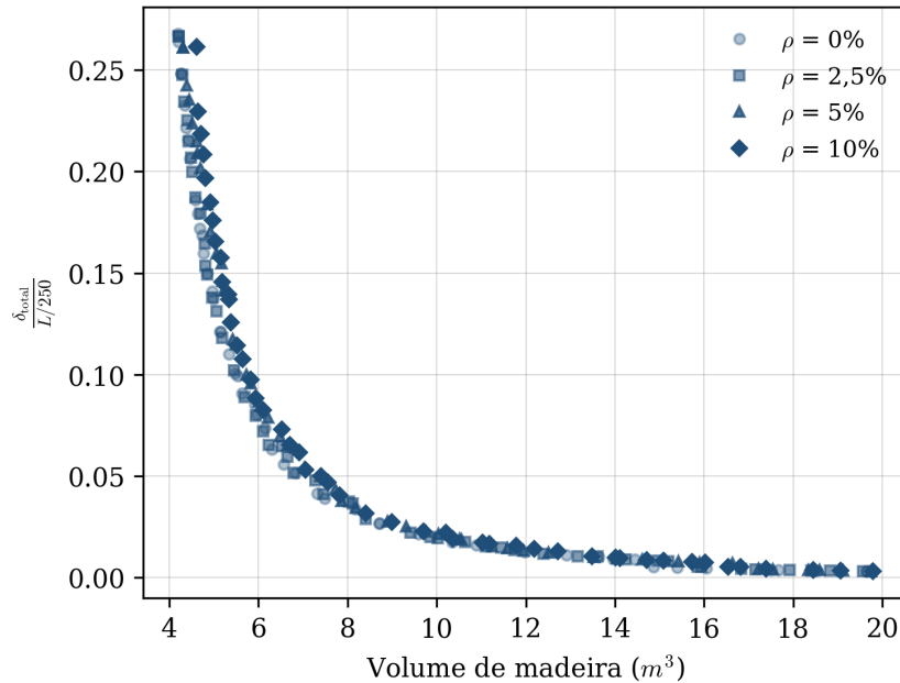
Figura 10: Fronteiras eficientes da célula C-13 para \rho = 0\% , 2,5%, 5% e 10%.
