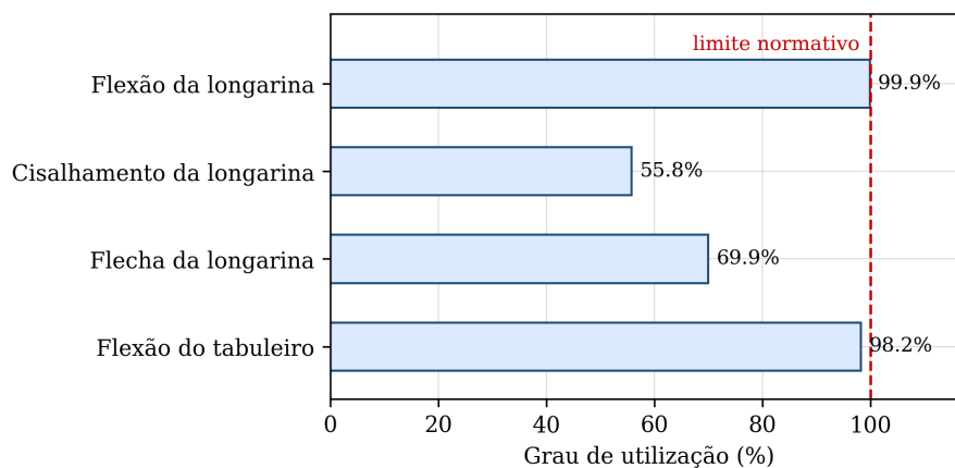
Figura 9: Grau de utilização de cada verificação normativa para a solução selecionada da fronteira robusta da célula C-13.
