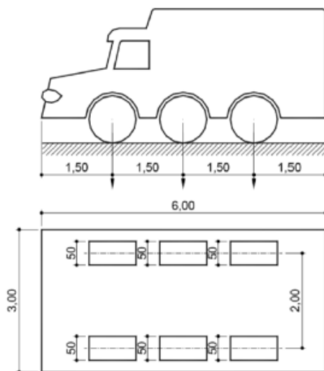
Figura 3: Configuração trem de tipo.
