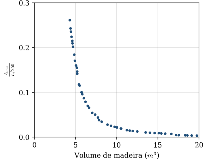
Figura 8: Fronteira eficiente da célula de referência C-13 ( L = 5,0 m, D40, \rho = 5\% ).
