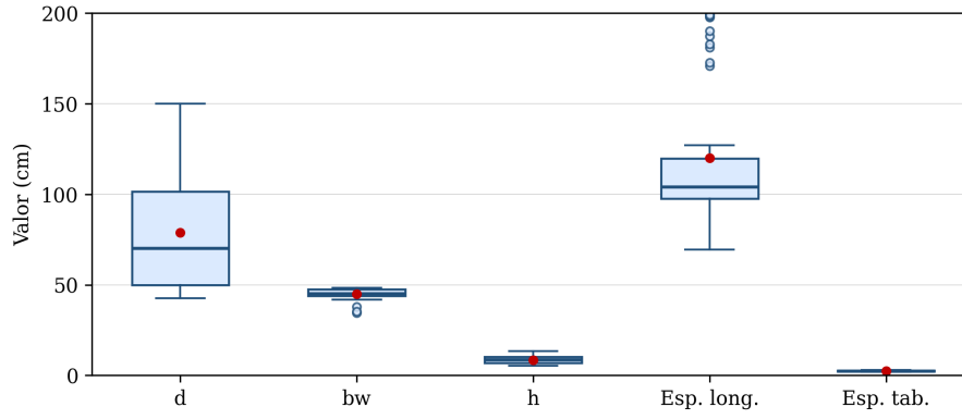
Figura 13: Dispersão das variáveis de projeto ao longo da fronteira eficiente da célula C-13.
