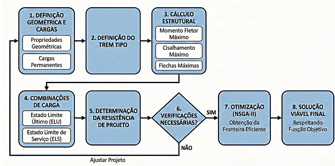
Figura 4: Fluxograma da otimização e análise do dimensionamento de pontes de madeira.
