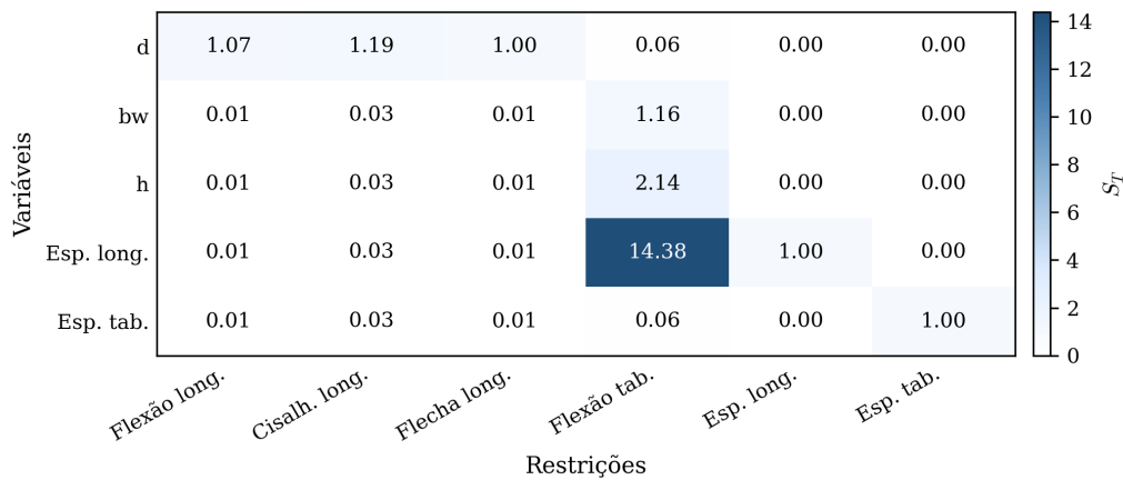
Figura 12: Índices de Sobol de efeito total ( S_{T_i} ) das variáveis de projeto sobre as restrições, célula C-13.
