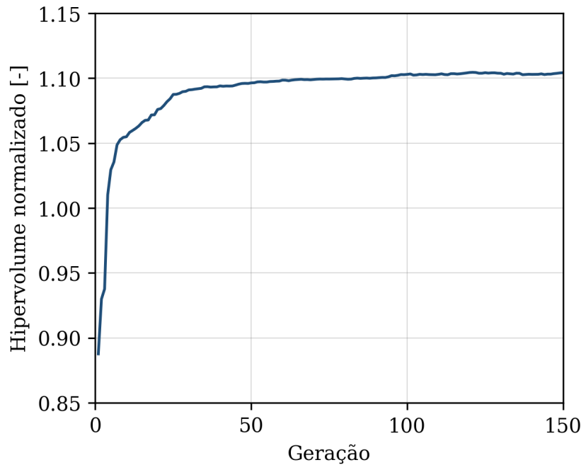
Figura 11: Evolução do hipervolume ao longo das gerações do NSGA-II.
