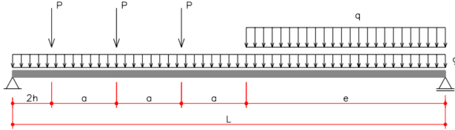
Figura 9.7 – Posicionamento do veículo-tipo para cortante
