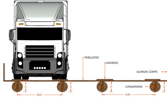
Figura 11: Representação conceitual do sistema estrutural da ponte de madeira.
