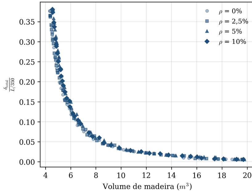
Figura 16: Fronteiras eficientes da célula C-13 para \rho = 0\% , 2,5%, 5% e 10%.
