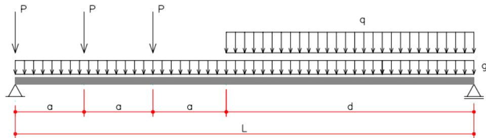
Figura 9.6 – Posicionamento do veículo-tipo para reação de apoio
