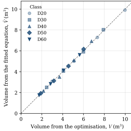
Figura 12: Volume estimado pela equação de pré-dimensionamento (Equação 33) contra o volume obtido na otimização, para as vinte células da matriz.
