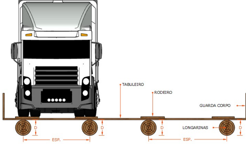
Figura 4: Representação conceitual do sistema estrutural da ponte de madeira.
