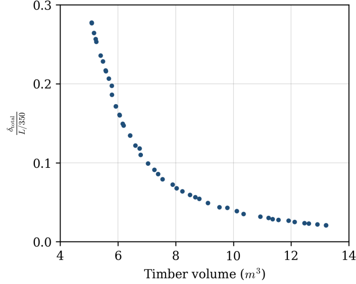
Figura 6: Fronteira eficiente da célula de referência C-13 ( L = 5,0 m, D40, \rho = 5\% ).
