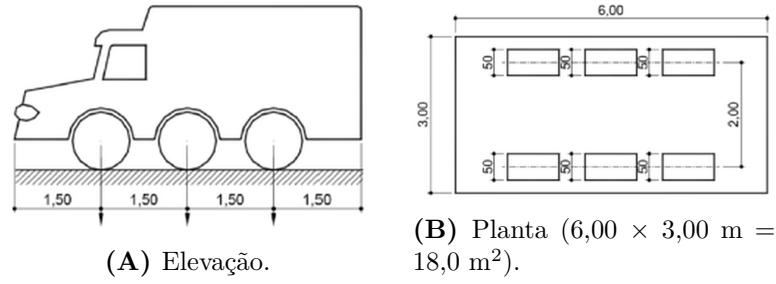
Figura 1: Configuração do trem-tipo TB-240 (NBR 7188, 2024).
