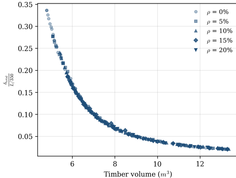
Figura 8: Fronteiras eficientes da célula C-13 para \rho = 0\% , 5%, 10%, 15% e 20%.
