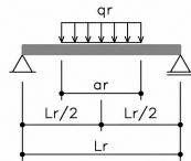
Figura 3: Posicionamento crítico de uma roda sobre o tabuleiro (Calil Júnior et al., 2006).
