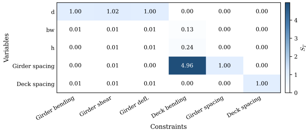
Figura 9: Índices de Sobol de efeito total ( S_{T_i} ) das variáveis de projeto sobre as restrições, célula C-13.
