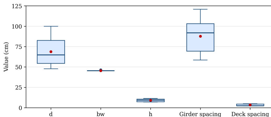
Figura 10: Dispersão das variáveis de projeto ao longo da fronteira eficiente da célula C-13.
