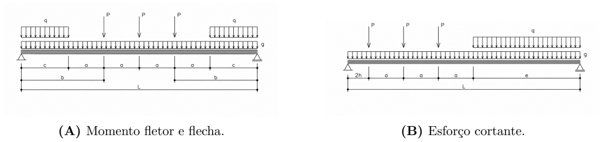
Figura 2: Posicionamento do veículo-tipo para o cálculo dos esforços na longarina (Calil Júnior et al., 2006).
