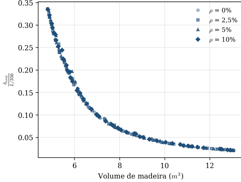
Figura 16: Fronteiras eficientes da célula C-13 para \rho = 0\% , 2,5\% , 5\% e 10\% .
