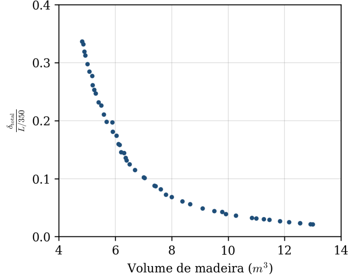
Figura 14: Fronteira eficiente da célula de referência C-13 ( L = 5,0 m, D40, \rho = 5\% ).
