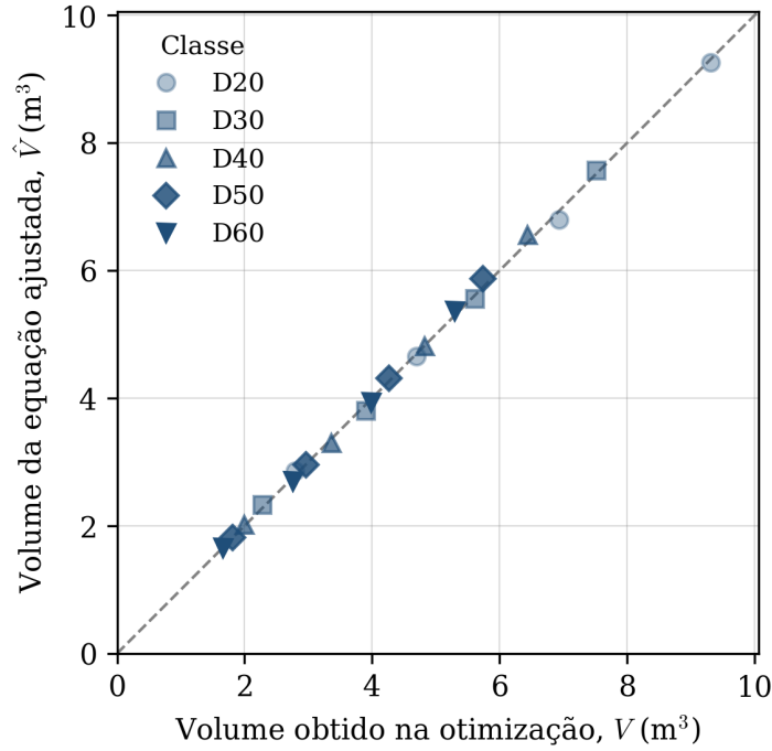
Figura 23: Volume estimado pela equação de pré-dimensionamento (Equação 45) contra o volume obtido na otimização, para as vinte células da matriz.
