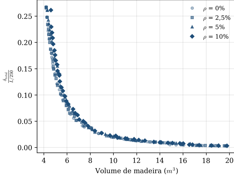
Figura 8: Fronteiras eficientes da célula C-13 para \rho = 0\% , 2,5\% , 5\% e 10\% .
