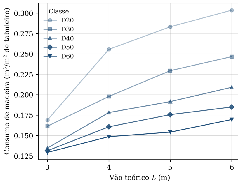
Figura 13: Consumo de madeira por metro quadrado de tabuleiro, em função do vão teórico, por classe de resistência.
