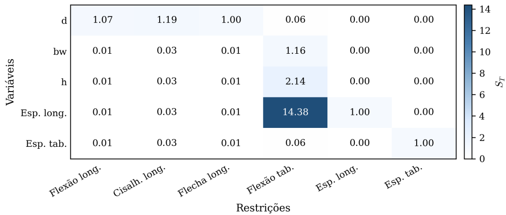
Figura 10: Índices de Sobol de efeito total ( S_{T_i} ) das variáveis de projeto sobre as restrições, célula C-13.
