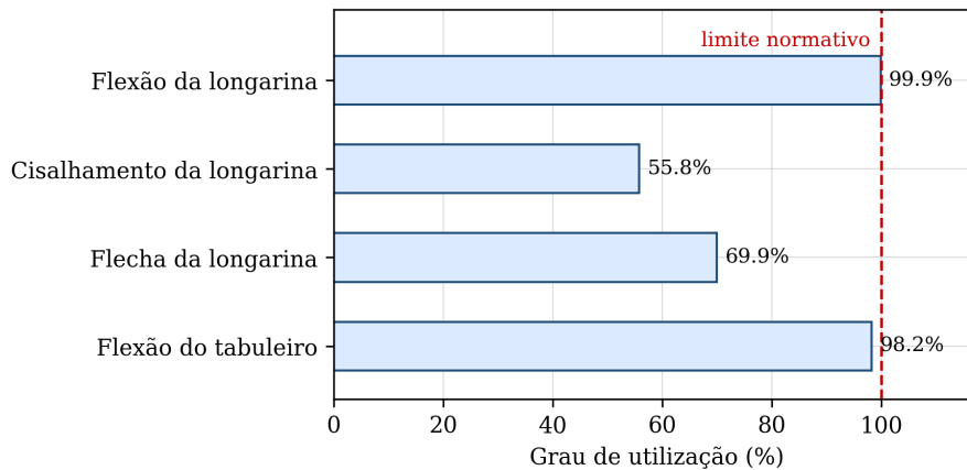
Figura 7: Grau de utilização de cada verificação normativa para a solução selecionada da fronteira robusta da célula C-13.
