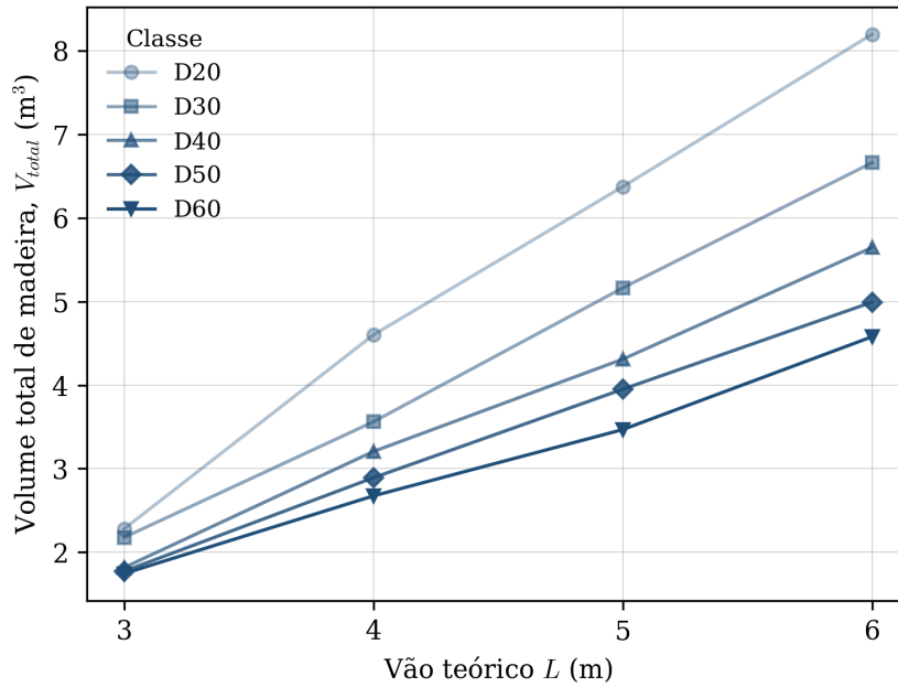
Figura 12: Volume total de madeira em função do vão teórico, por classe de resistência.
