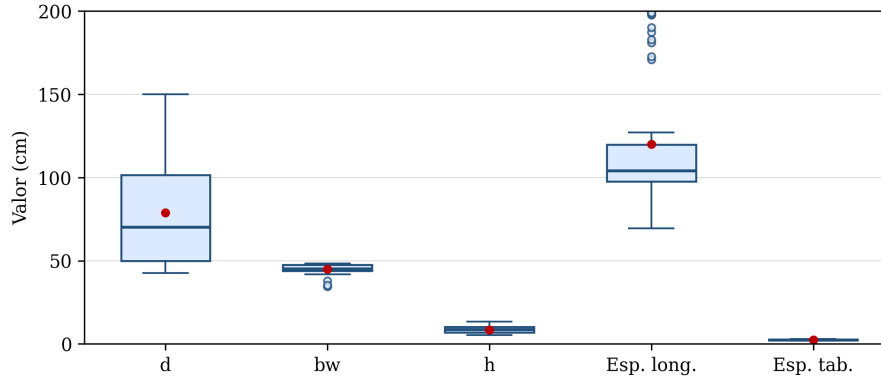
Figura 11: Dispersão das variáveis de projeto ao longo da fronteira eficiente da célula C-13.
