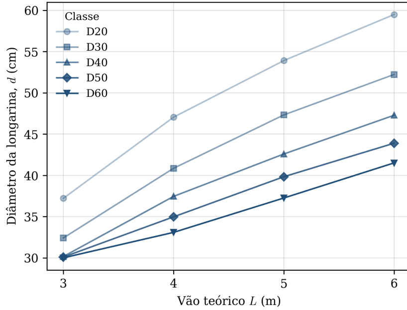
Figura 14: Diâmetro de longarina requerido em função do vão teórico, por classe de resistência.
