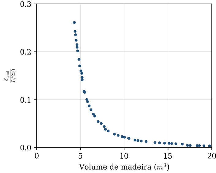
Figura 6: Fronteira eficiente da célula de referência C-13 ( L = 5,0 m, D40, \rho = 5\% ).
