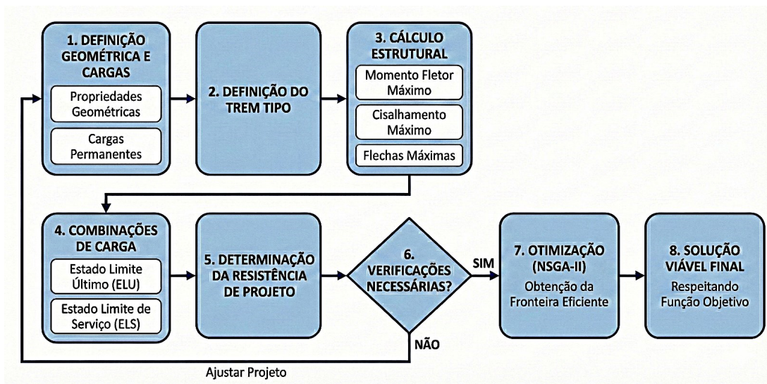
Figura 5: Fluxograma da otimização e análise do dimensionamento de pontes de madeira.
