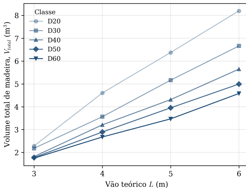
Figura 15: Volume total de madeira em função do vão teórico, por classe de resistência.
