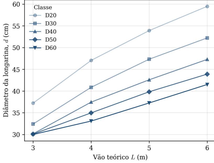
Figura 17: Diâmetro de longarina requerido em função do vão teórico, por classe de resistência.
