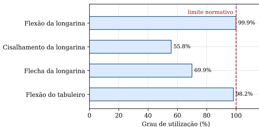
Figura 10: Grau de utilização de cada verificação normativa para a solução selecionada da fronteira robusta da célula C-13.
