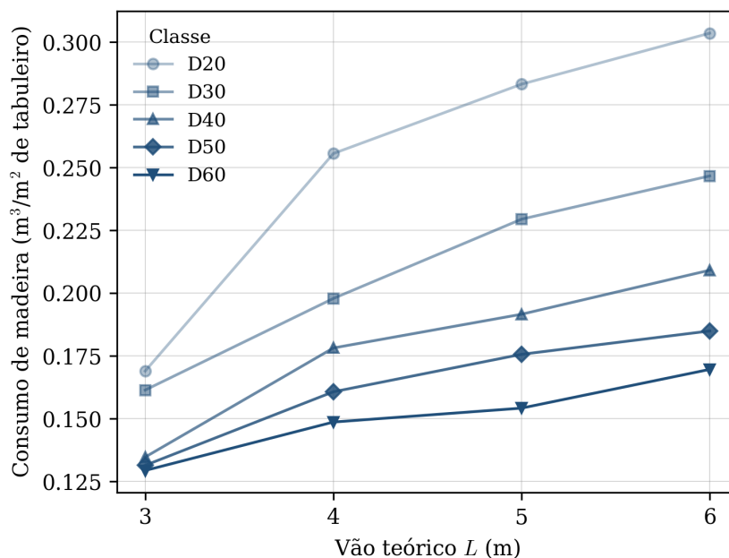
Figura 16: Consumo de madeira por metro quadrado de tabuleiro, em função do vão teórico, por classe de resistência.
