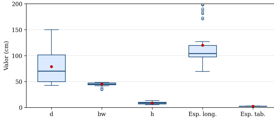
Figura 14: Dispersão das variáveis de projeto ao longo da fronteira eficiente da célula C-13.
