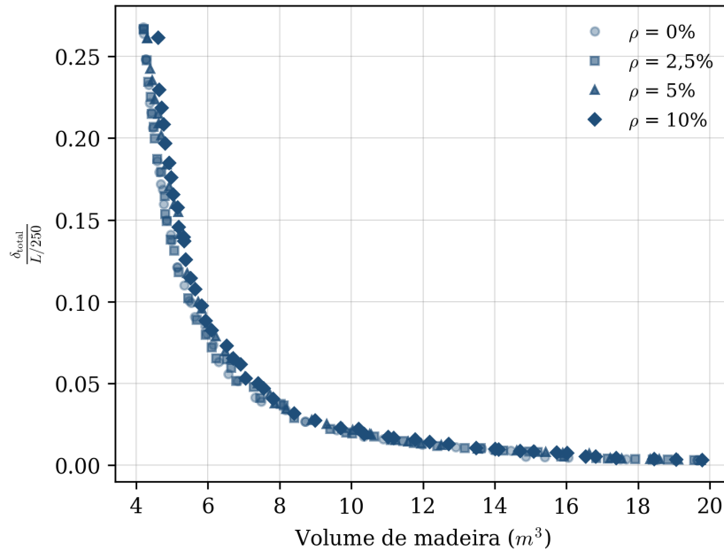
Figura 11: Fronteiras eficientes da célula C-13 para \rho = 0\% , 2,5%, 5% e 10%.
