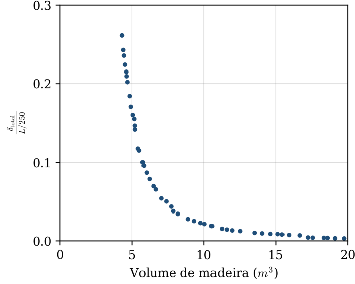
Figura 9: Fronteira eficiente da célula de referência C-13 ( L = 5,0 m, D40, \rho = 5\% ).
