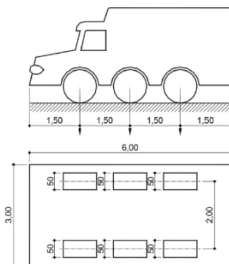
Figura 4: Configuração trem de tipo.
