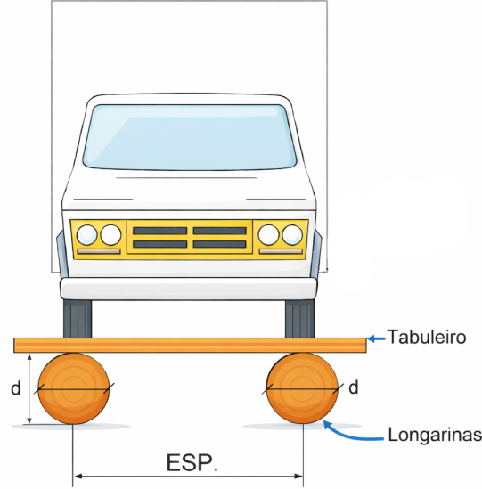
Figura 6: Representação conceitual do sistema estrutural da ponte de madeira.
