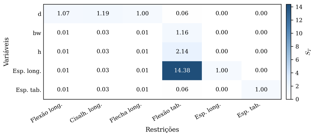
Figura 13: Índices de Sobol de efeito total ( S_{T_i} ) das variáveis de projeto sobre as restrições, célula C-13.
