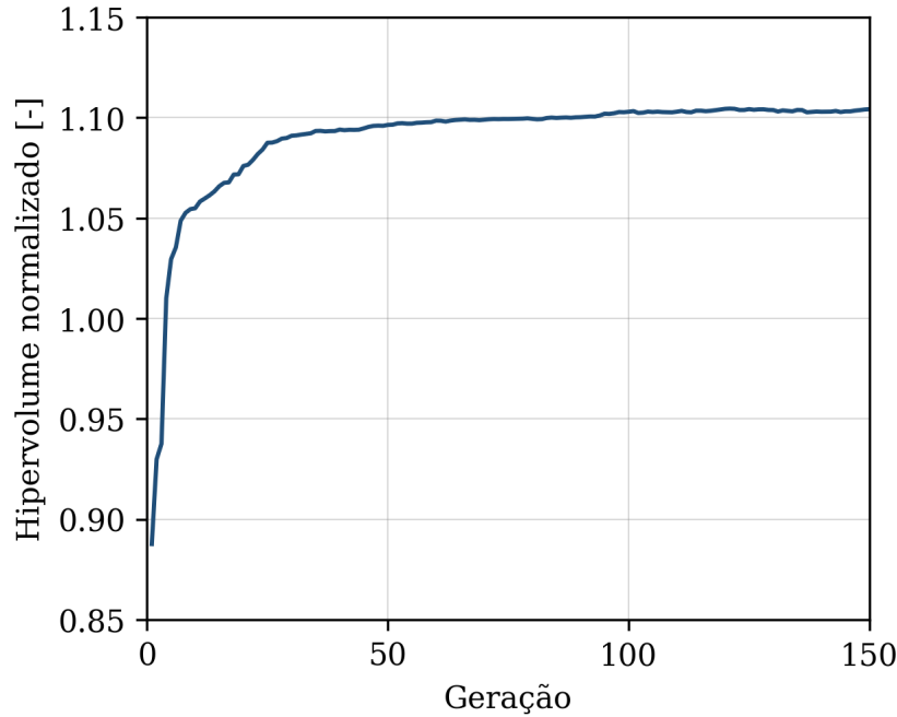
Figura 12: Evolução do hipervolume ao longo das gerações do NSGA-II.
