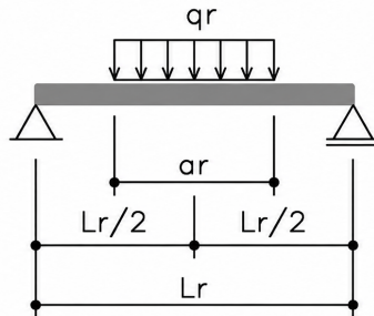
Figura 4: Posicionamento crítico de uma roda sobre o tabuleiro (Calil Júnior et al., 2006).
