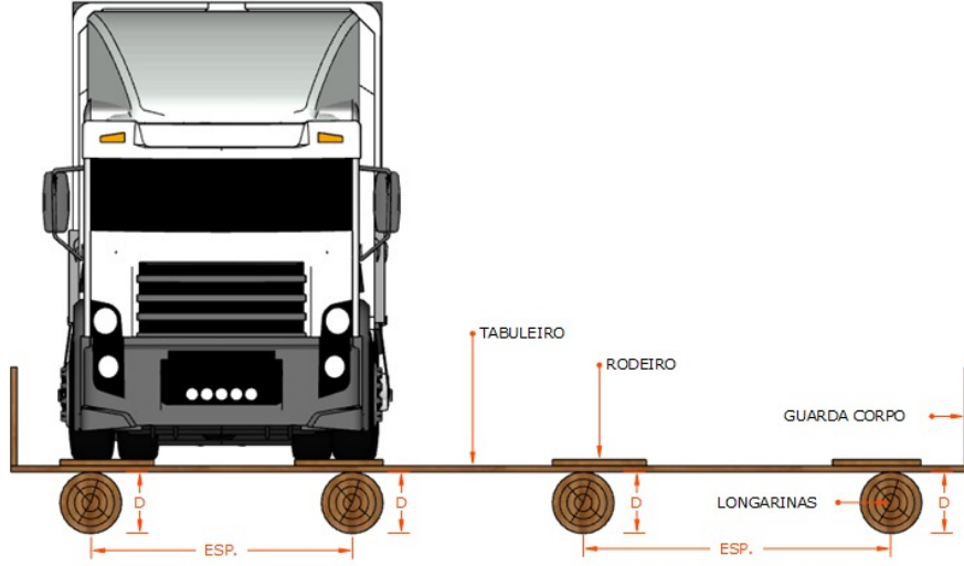
Figura 5: Representação conceitual do sistema estrutural da ponte de madeira.
