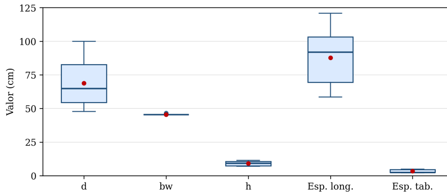
Figura 12: Dispersão das variáveis de projeto ao longo da fronteira eficiente da célula C-13.
