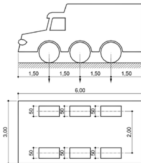
Figura 2: Configuração trem de tipo (NBR 7188, 2024).
