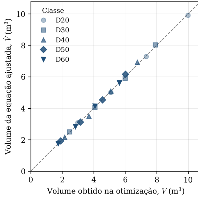
Figura 14: Volume estimado pela equação de pré-dimensionamento (Equação 42) contra o volume obtido na otimização, para as vinte células da matriz.
