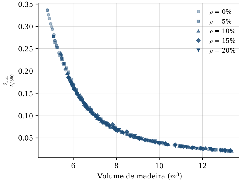
Figura 10: Fronteiras eficientes da célula C-13 para \rho = 0\% , 5\% , 10\% , 15\% e 20\% .
