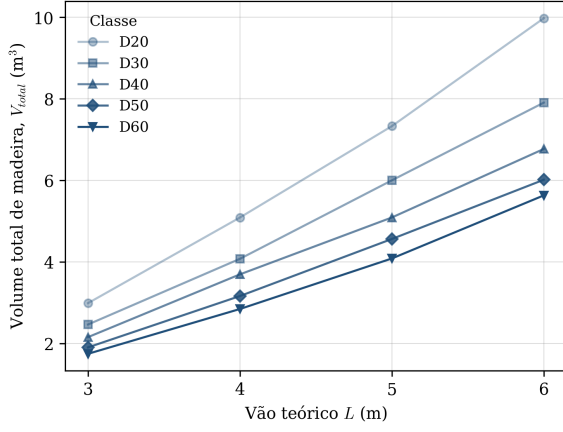
(A) Volume total de madeira em função do vão teórico.
