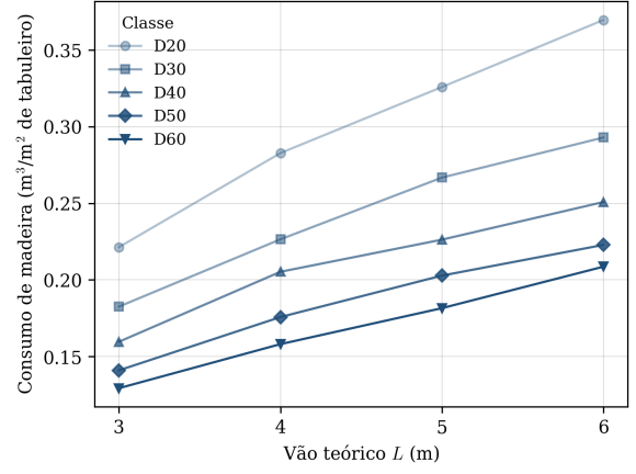
(B) Consumo de madeira por metro quadrado de tabuleiro.
