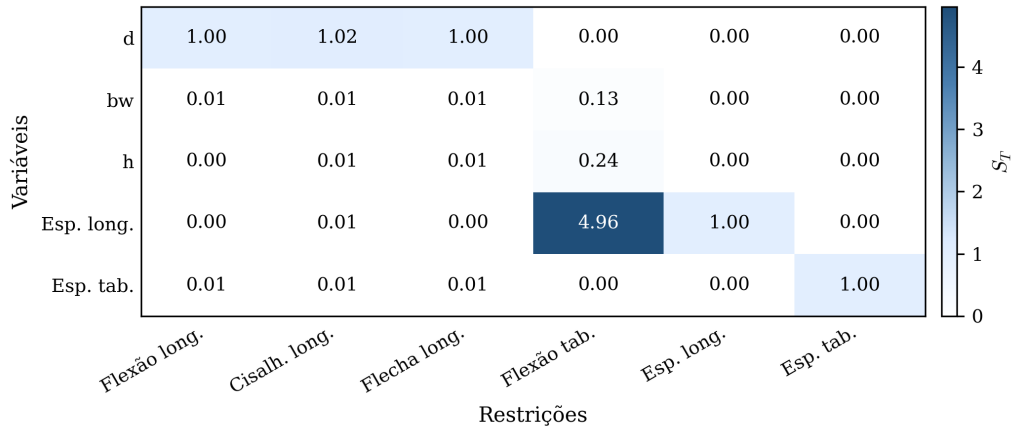
Figura 11: Índices de Sobol de efeito total ( S_{T_i} ) das variáveis de projeto sobre as restrições, célula C-13.
