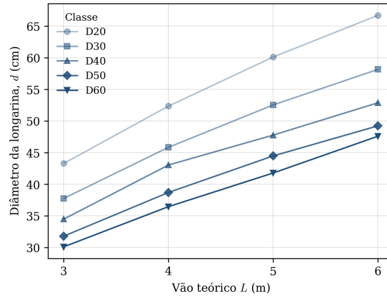
(C) Diâmetro de longarina requerido em função do vão teórico.
