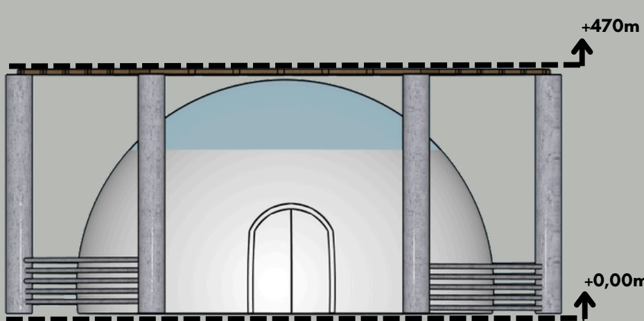
ELEWACJA Z PRZODU SKALA 1:100
