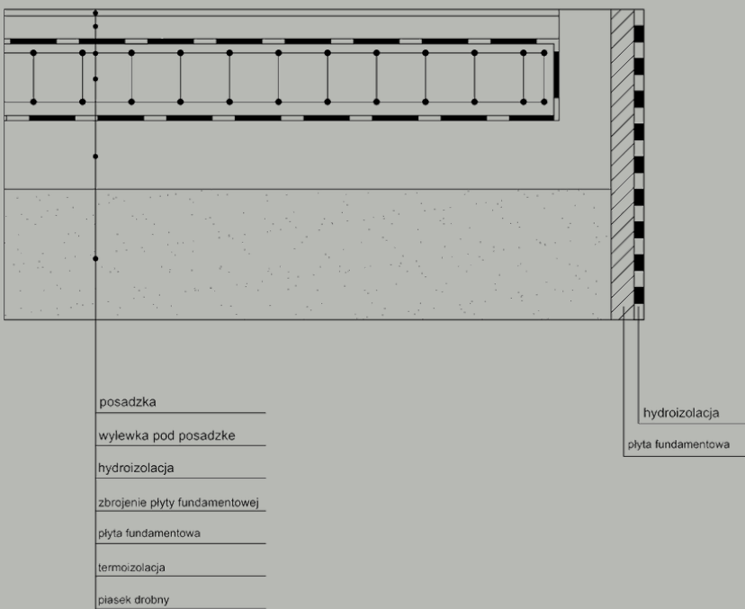
DETAL D1 SKALA 1:20
