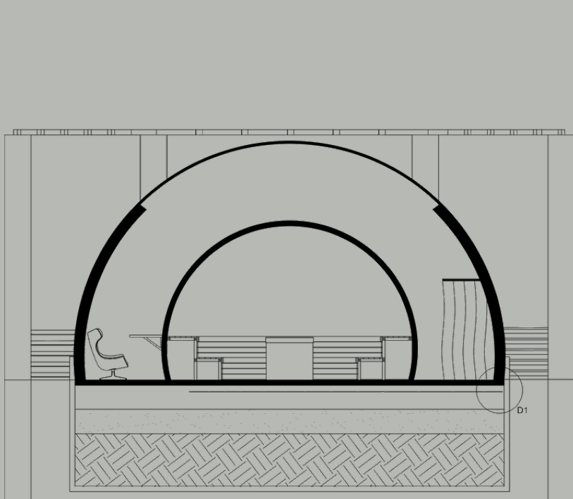
PRZEKRÓJ A-A' SKALA 1:100
