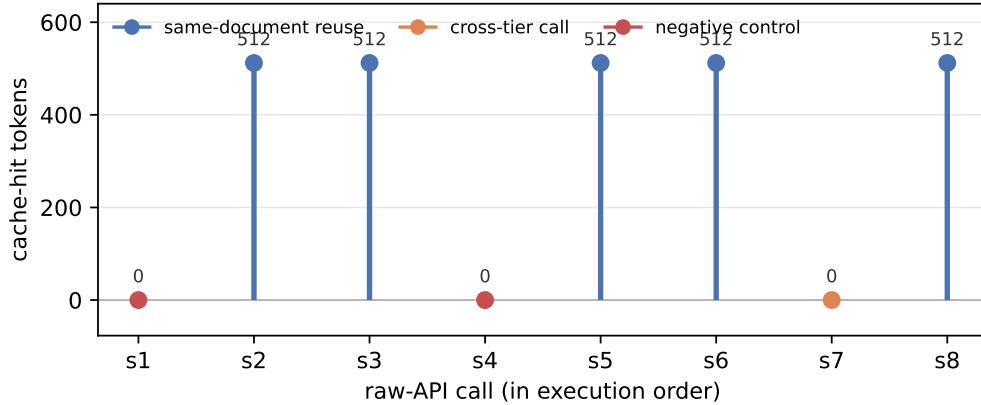
图 1: 通道 B 逐次调用的缓存命中 token 数（圆点落在 0 上表示该次调用零命中）。蓝色：同文档复用；橙色：跨层级调用；红色：负对照（首次调用尚无缓存、异文档基线）。
