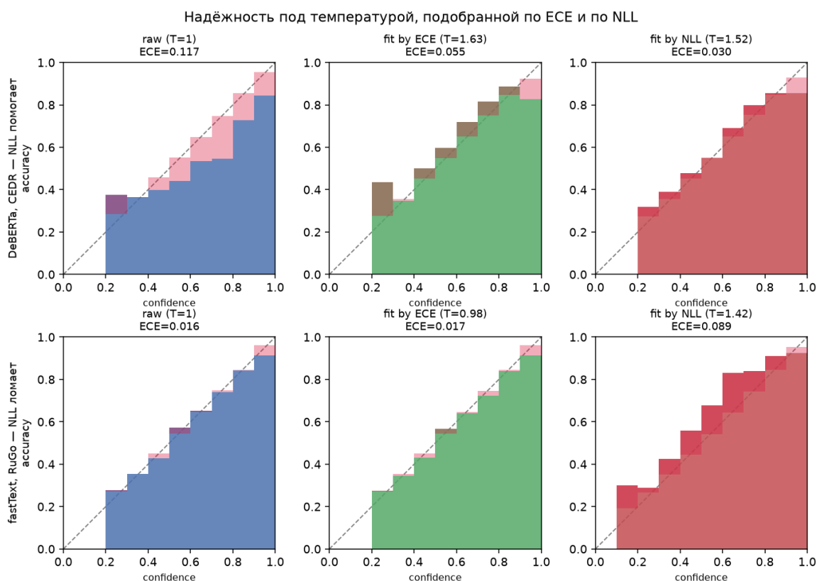
Рис. 3.4 – Диаграммы надёжности под температурой, подобранной по ECE и по NLL (синяя/зелёная заливка – ассигасу по бинам уверенности, розовое – разрыв до диагонали).
