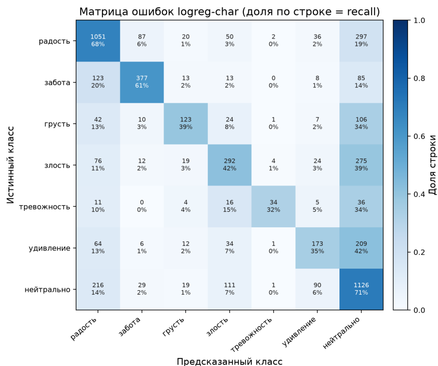
Рис. 3.6 – Матрица ошибок logreg-char (7 классов), нормированная по строкам: цвет – доля истинного класса (recall), число в ячейке – количество сообщений.
