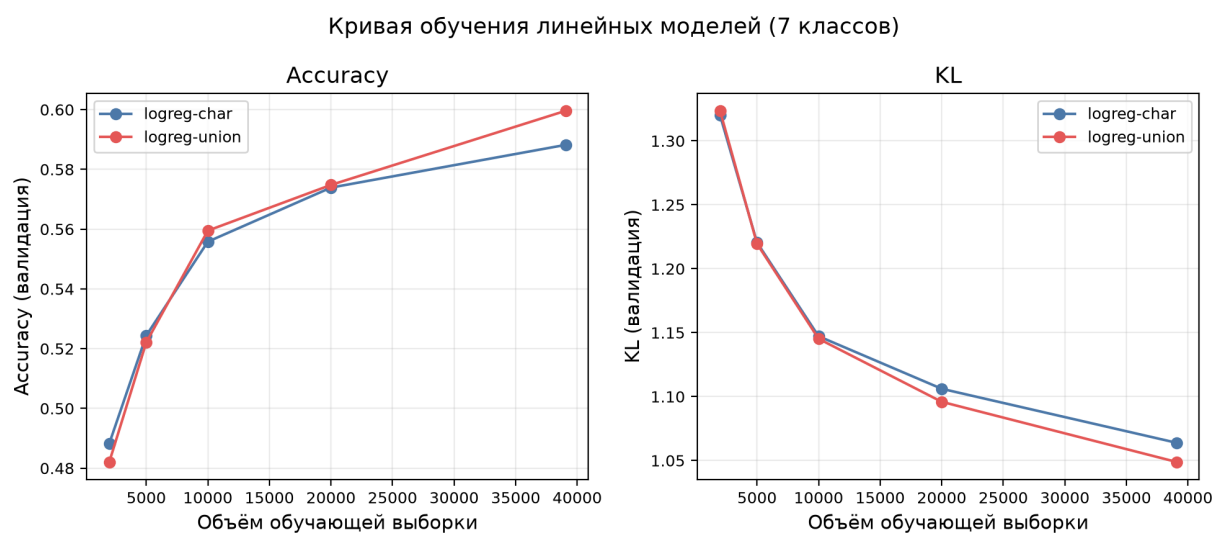
Рис. 3.7 – Кривая обучения линейных моделей: ассигасу и KL на валидации в зависимости от объёма обучающей выборки (7 классов).
