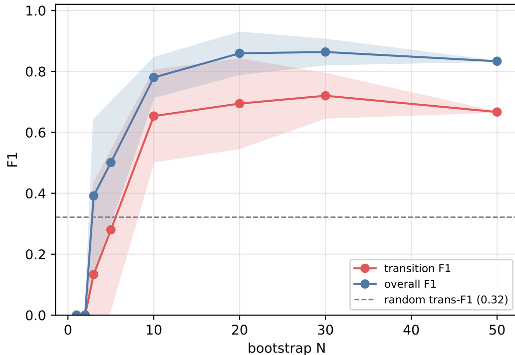
F1 vs bootstrap N
