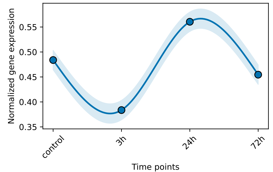
Start:LMPPs, CL: 34_0 (N=294)
