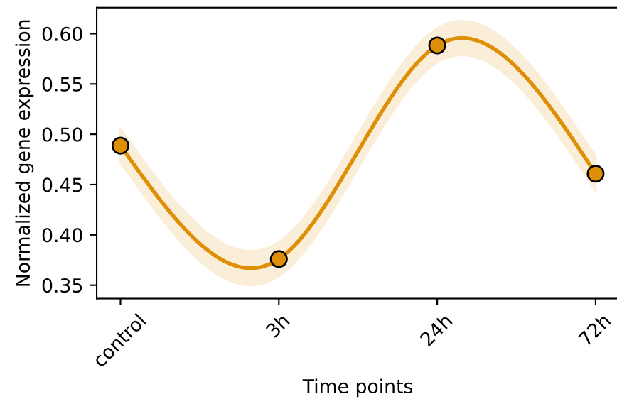
Start:LMPPs, CL: 35_0 (N=280)
