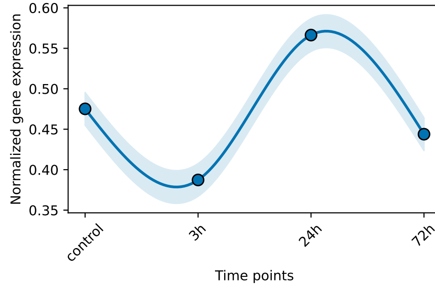
Start:MYP, CL: 37_0 (N=387)
