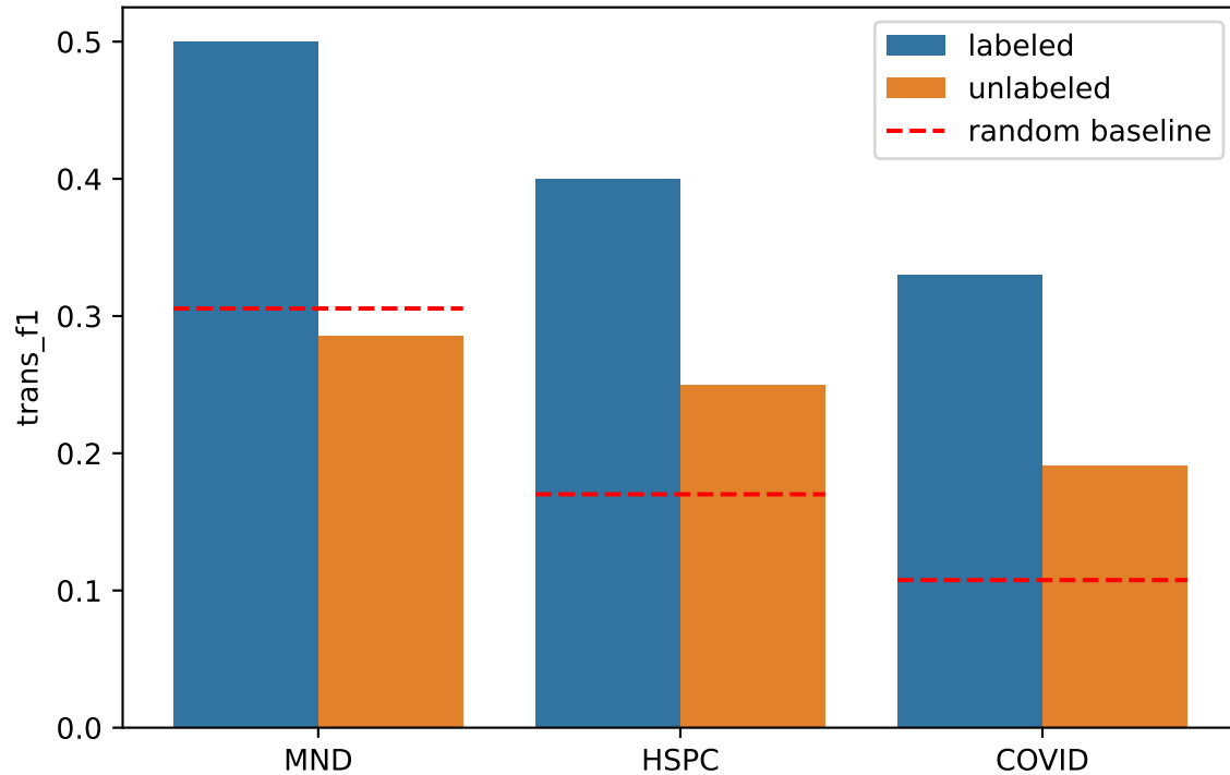
Transition-edge F1 (off-diagonal)
