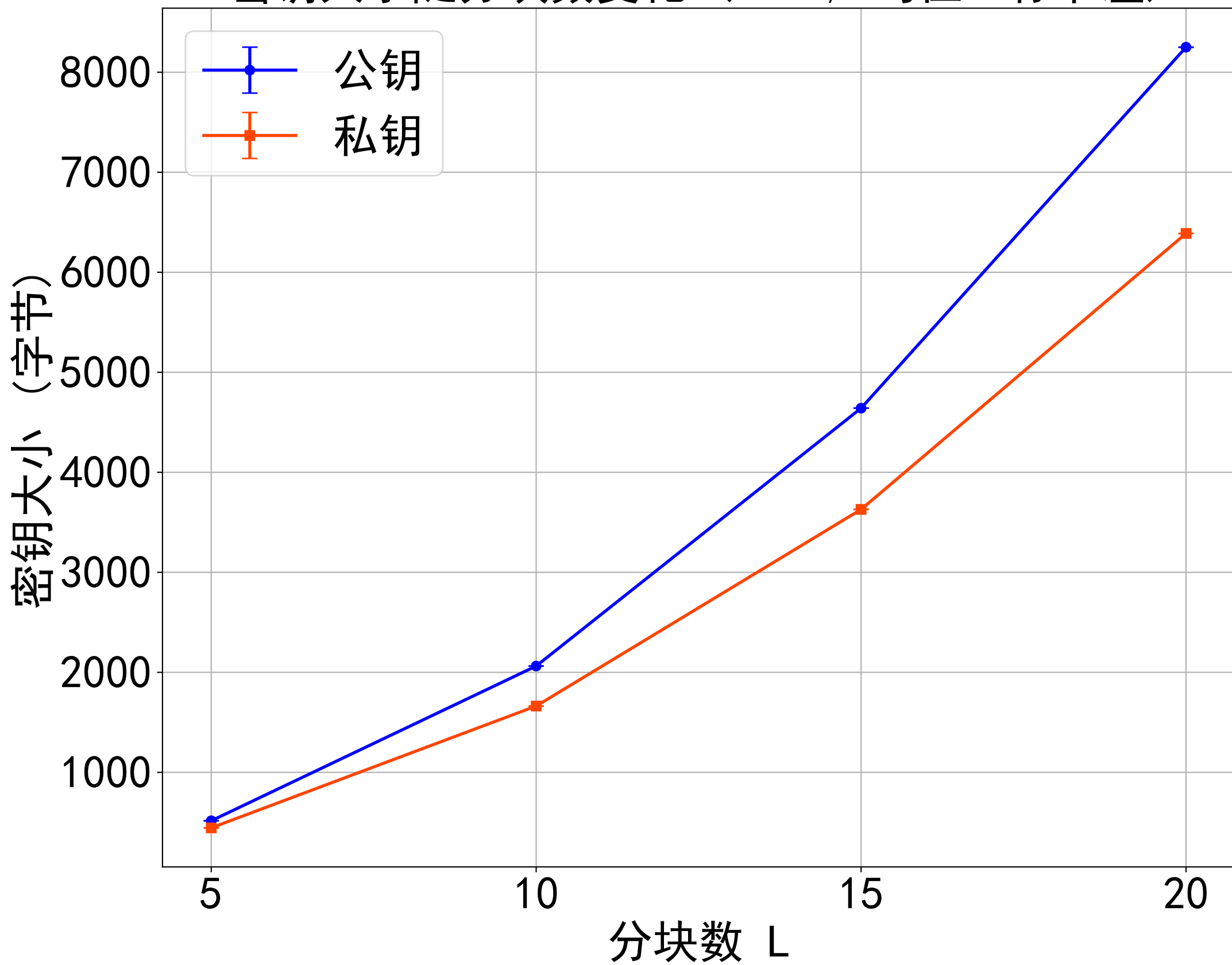
密钥大小随分块数变化 ( t_0=1 , 均值 \pm 标准差)
