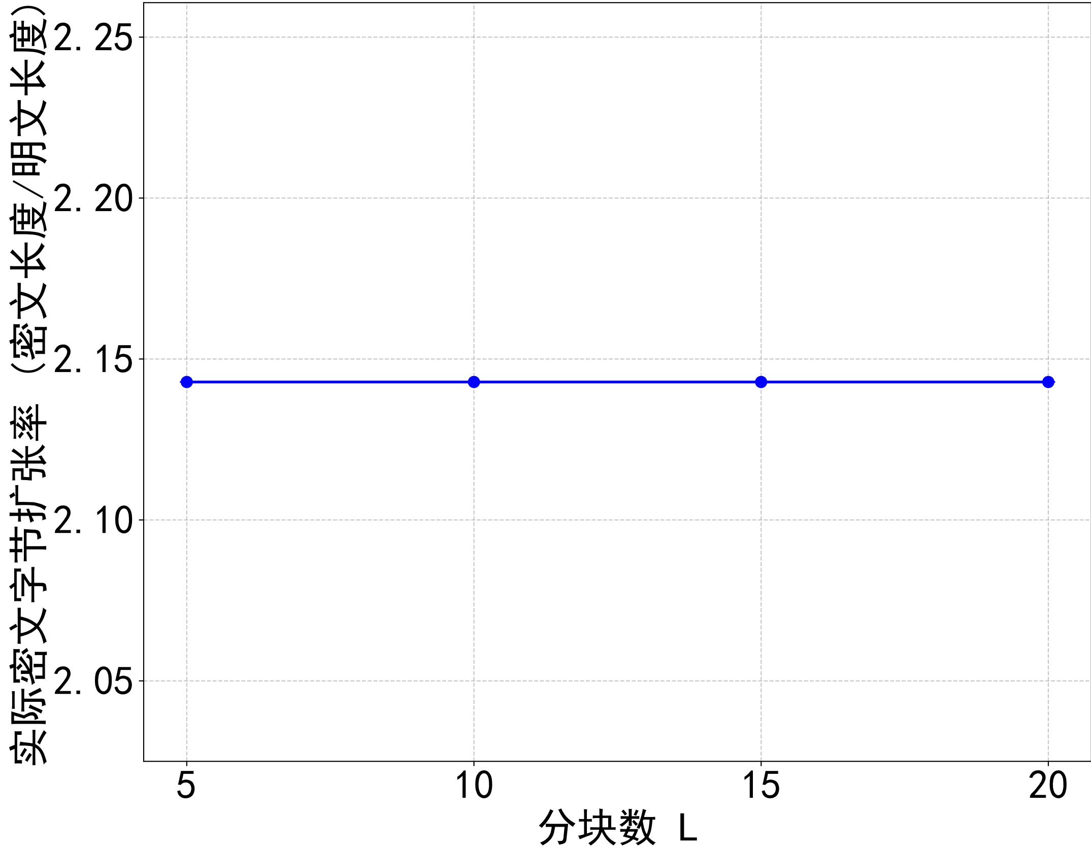
密文扩张率随分块数变化 (t0=2)
