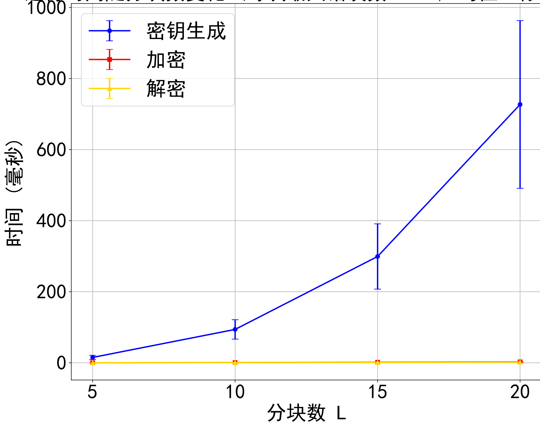
运行时间随分块数变化 (每块最大错误数 t_0=2 , 均值 \pm 标准差)
