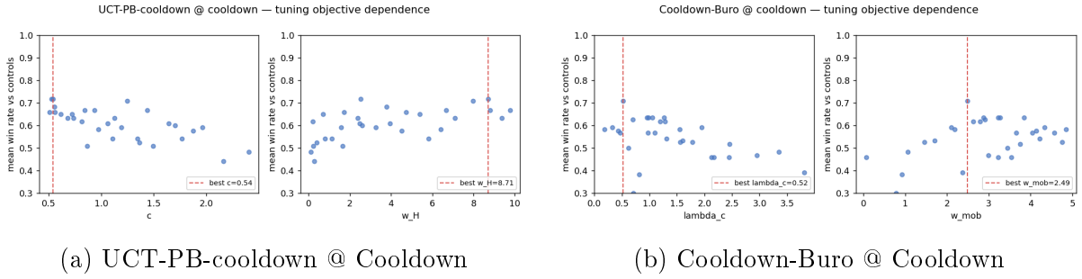
Rysunek 7: Zależność celu od hiperparametrów dla wybranych metod (PDP/slice). Dla PB-cooldown widać realną zależność od c i w_H ; dla heurystyki Buro funkcja jest płaska względem w_{mob} (parametr słabo ograniczony).
