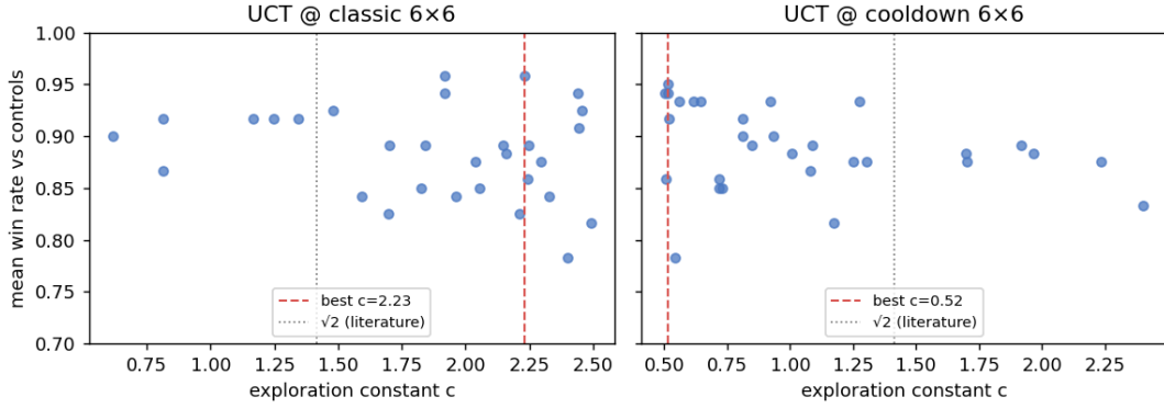
Rysunek 6: Zależność współczynnika wygranych UCT od stałej eksploracji c (wykres PDP/slice).
