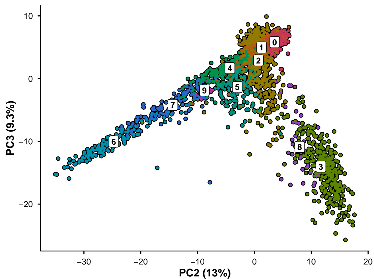
PC2 vs PC3
