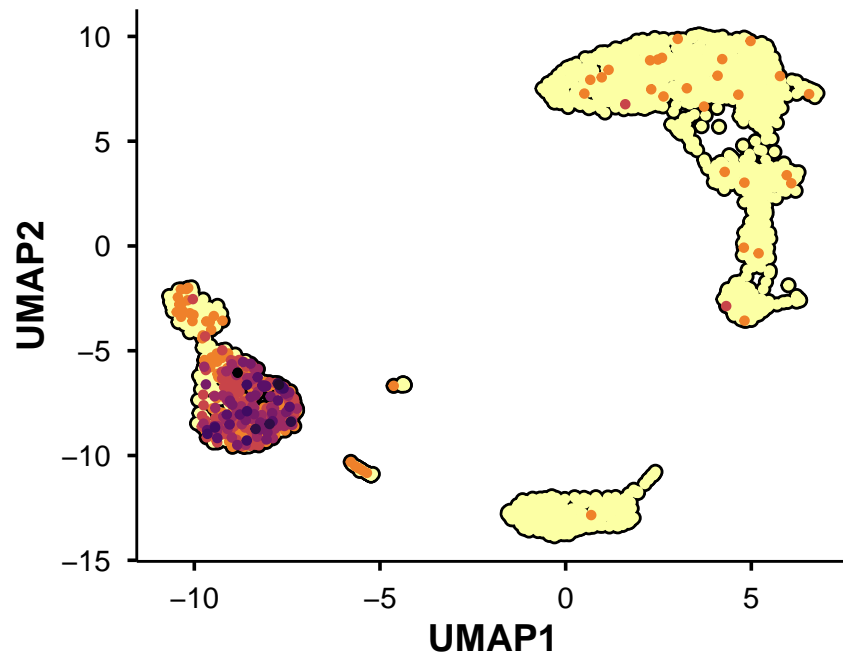
CD14
