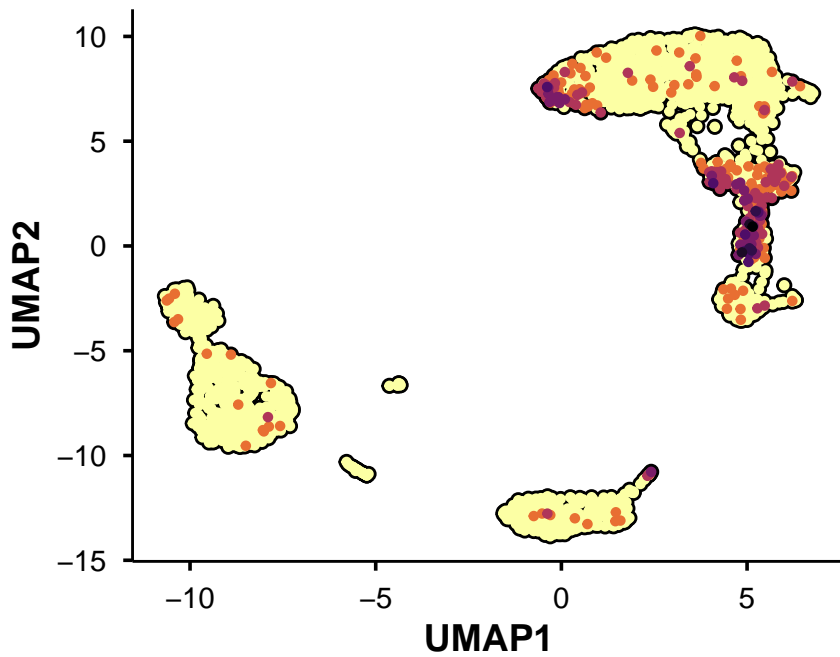
CD8A
