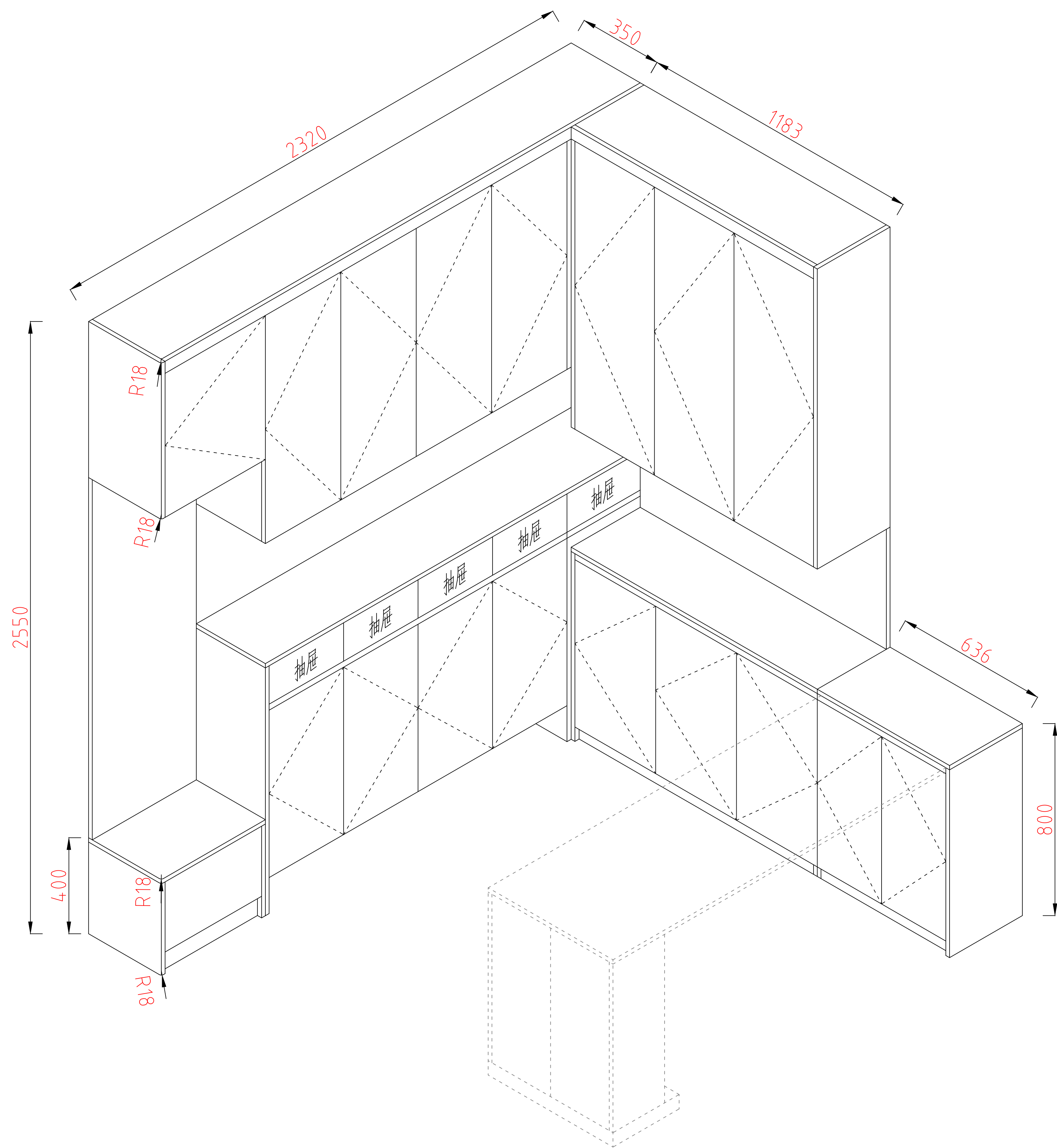
C字柜+工作台伸缩桌外观图
