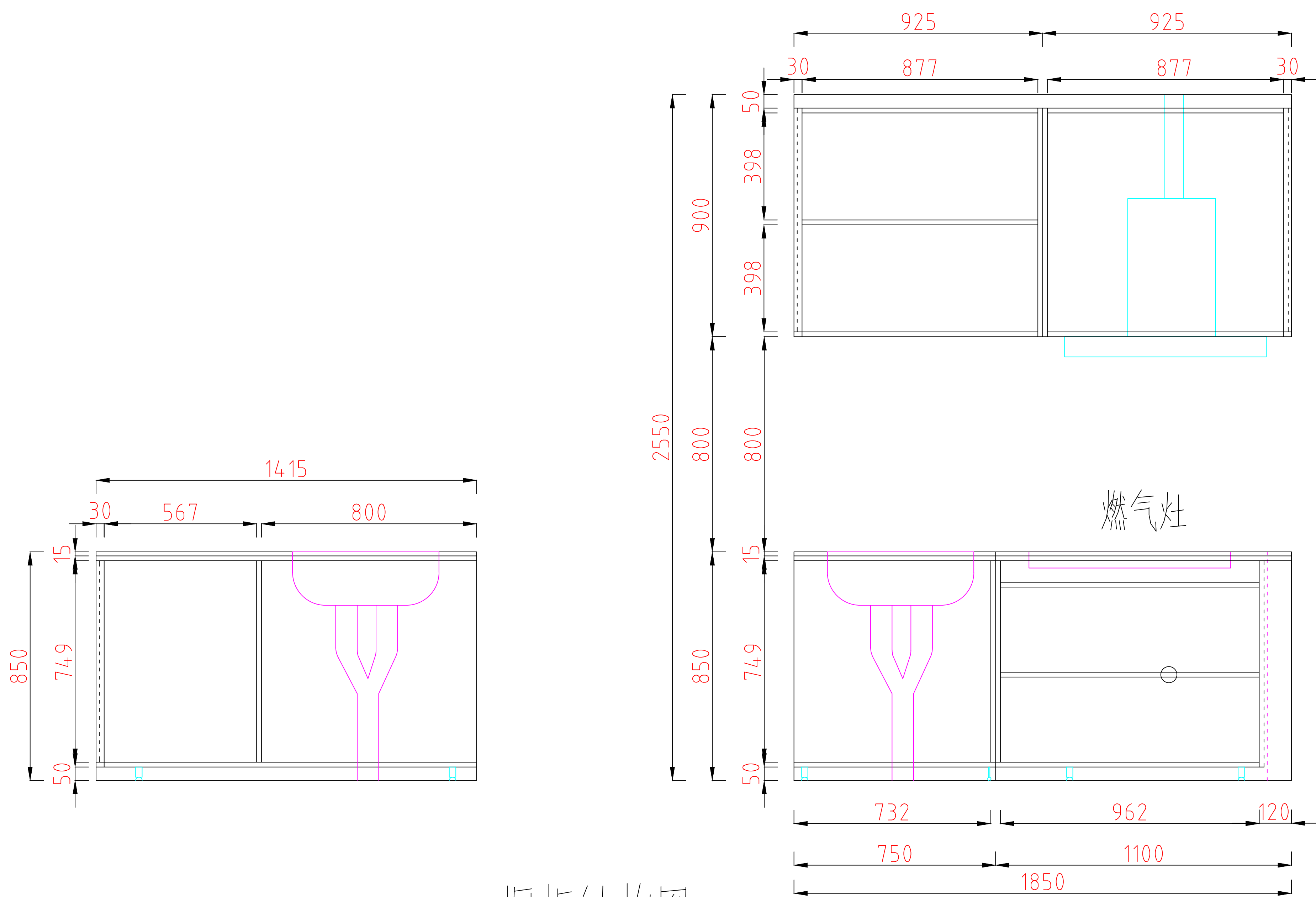
橱柜结构图
