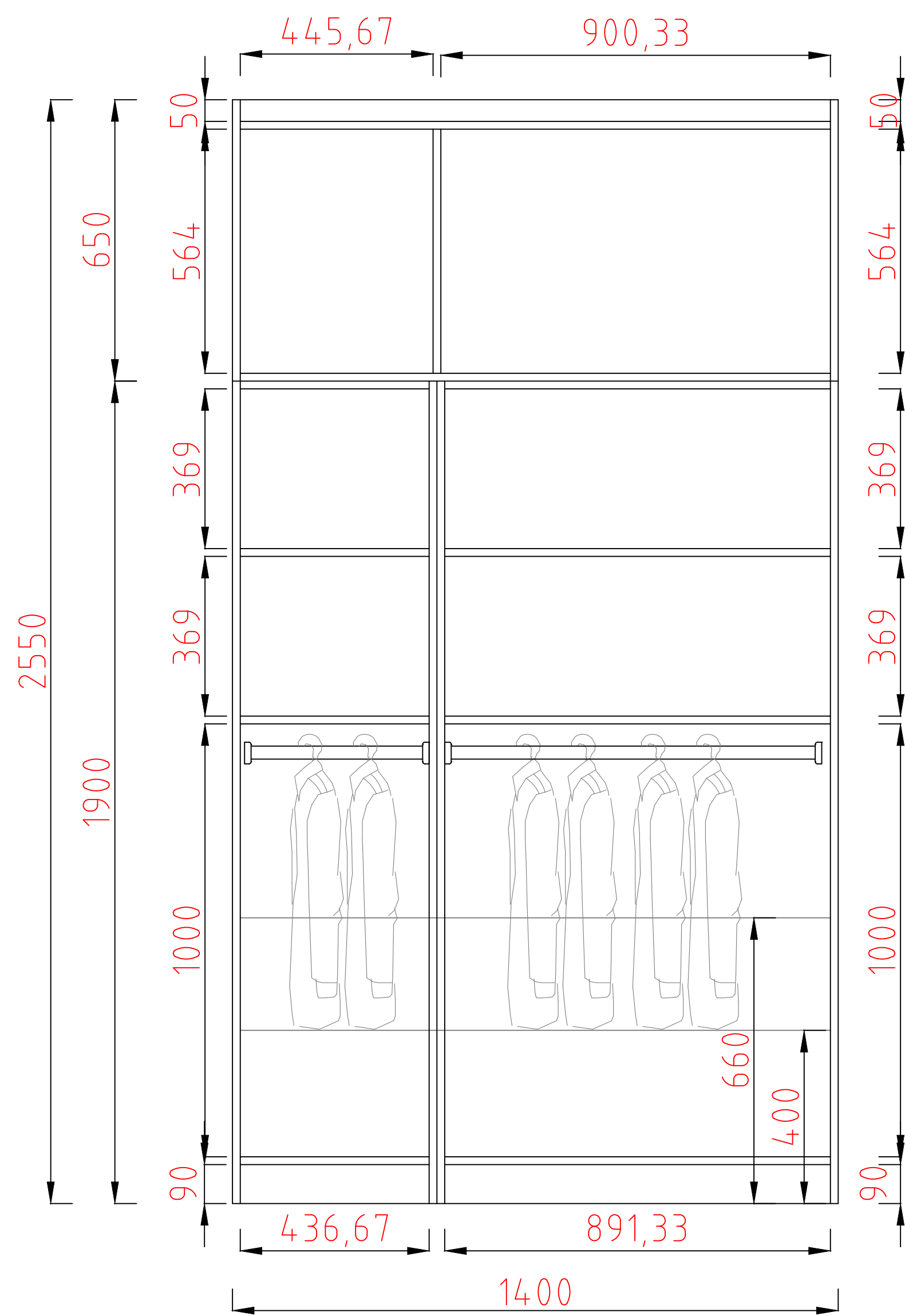
衣柜结构图
