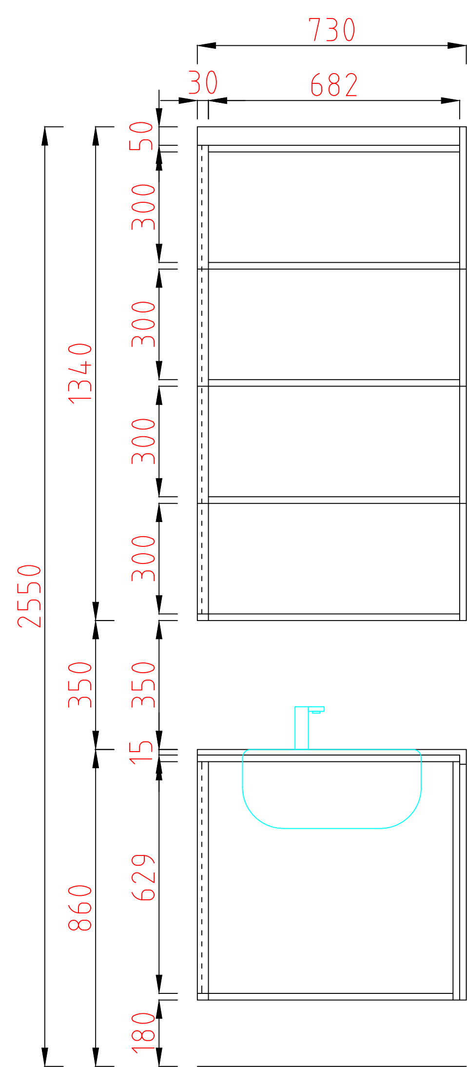
浴室柜结构图
