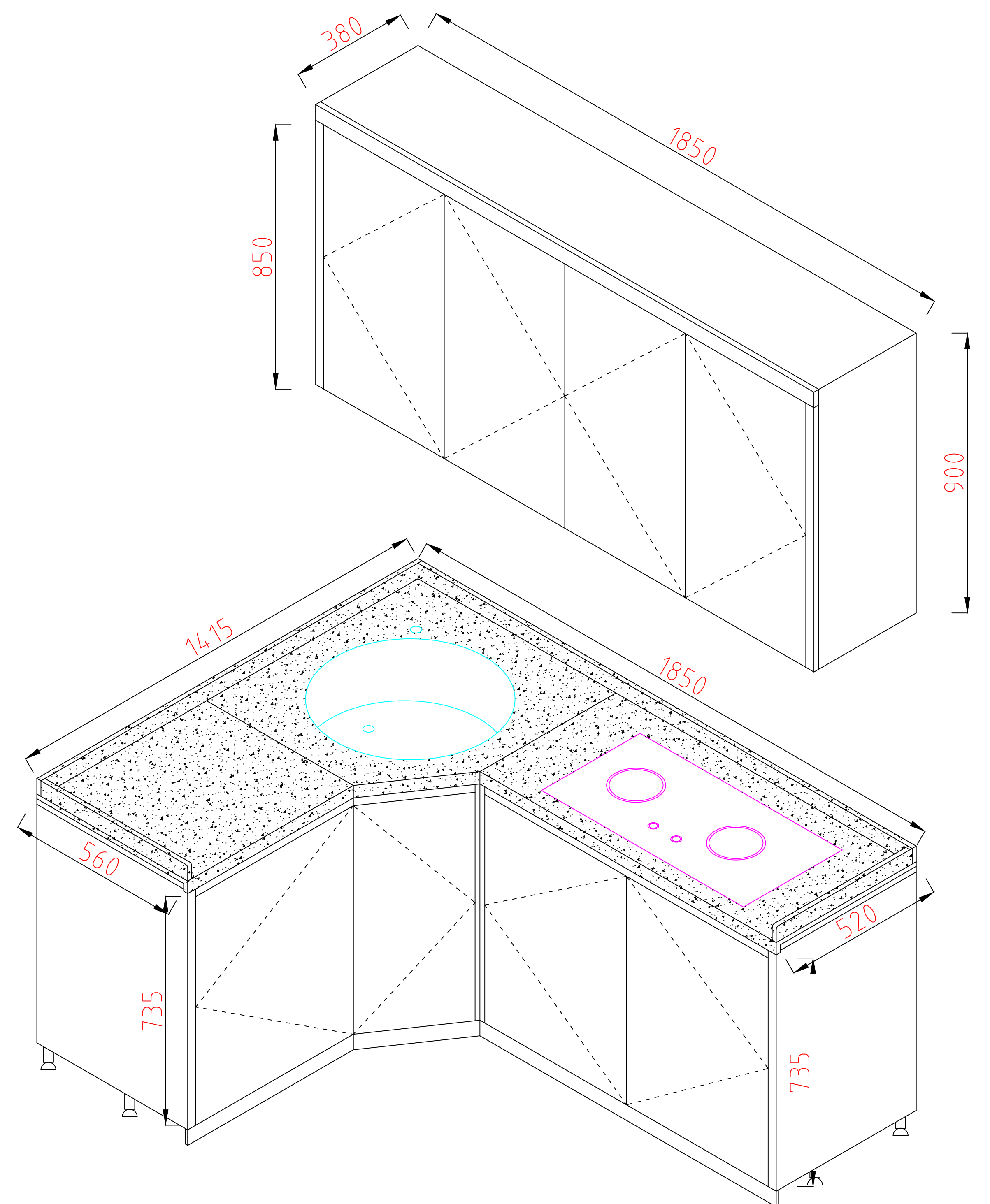
橱柜外观图
