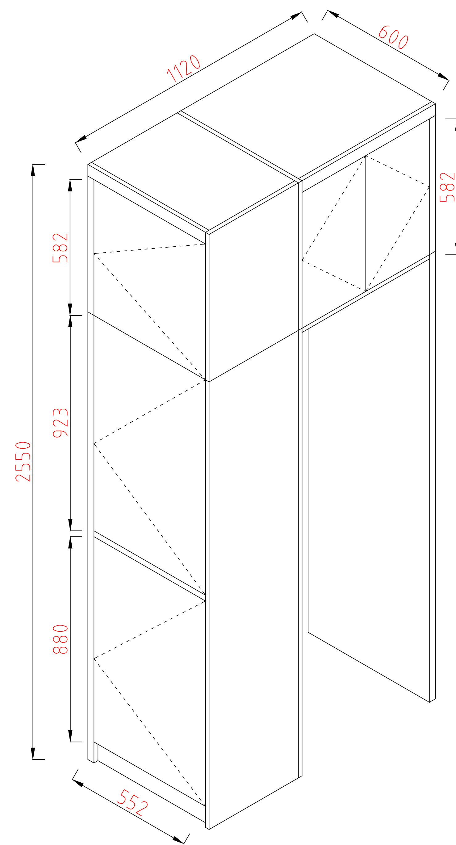
雪柜外观图
