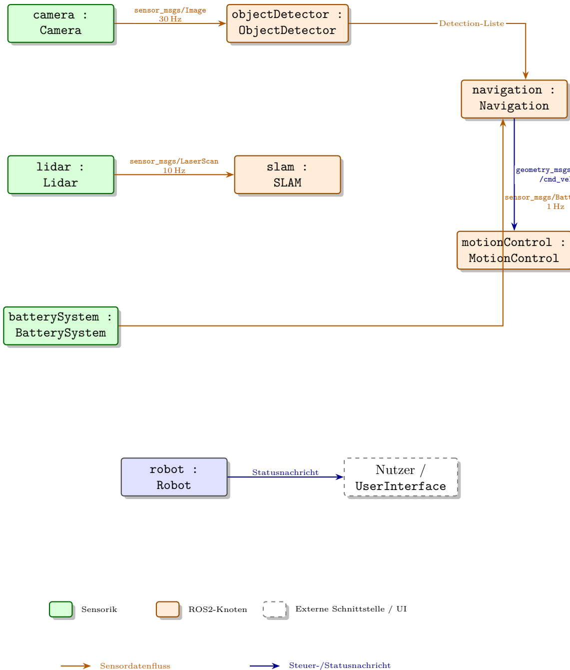
Figure 10.1: Schnittstellenübersicht des Indoor-Roboters: Sensordaten (orange) fließen über ObjectDetector und SLAM zur Navigation, Steuer- und Statusnachrichten (blau) verbinden Navigation, MotionControl und die Bedienoberfläche.
