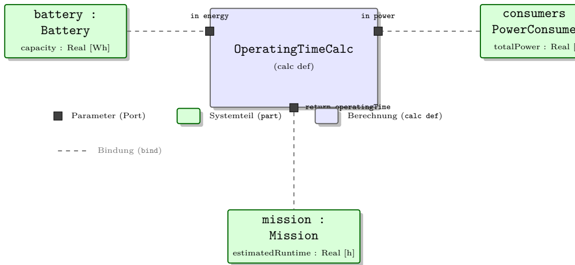
Figure 13.3: Parametrisches Diagramm zur Berechnung der Betriebszeit: OperatingTimeCalc verbindet die Batteriekapazität und die Leistungsaufnahme der Verbraucher zur geschätzten Laufzeit der Mission.
