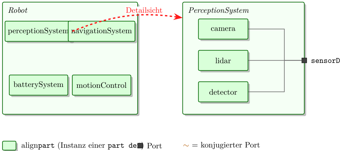
Figure 3.2: Struktursicht von Robot mit seinen Subsystemen und Detailsicht des PerceptionSystem mit Port sensorData.
