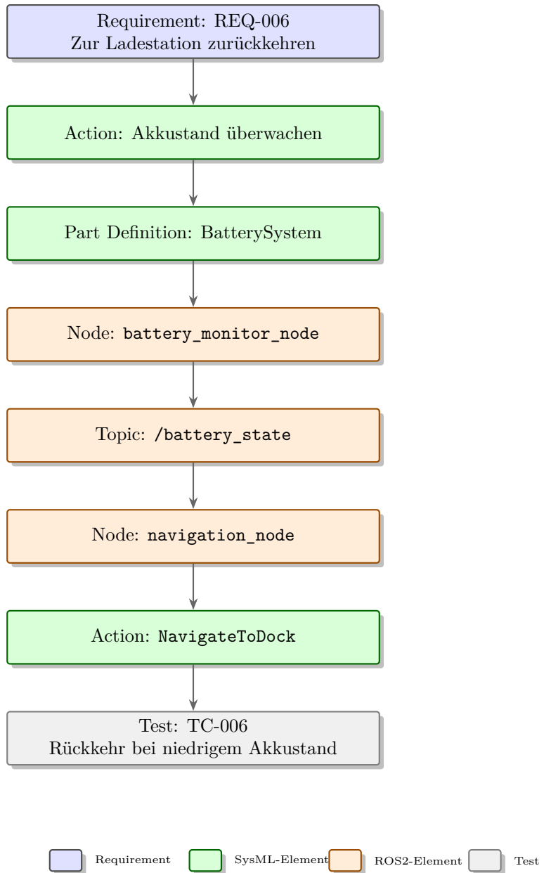
Figure 16.2: Traceability-Kette vom Requirement REQ-006 über SysML- und ROS2-Elemente bis zum Testfall TC-006.
