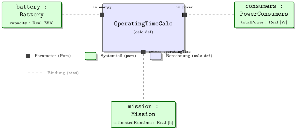
Figure 13.3: Parametrisches Diagramm zur Berechnung der Betriebszeit: OperatingTimeCalc verbindet die Batteriekapazität und die Leistungsaufnahme der Verbraucher zur geschätzten Laufzeit der Mission.
