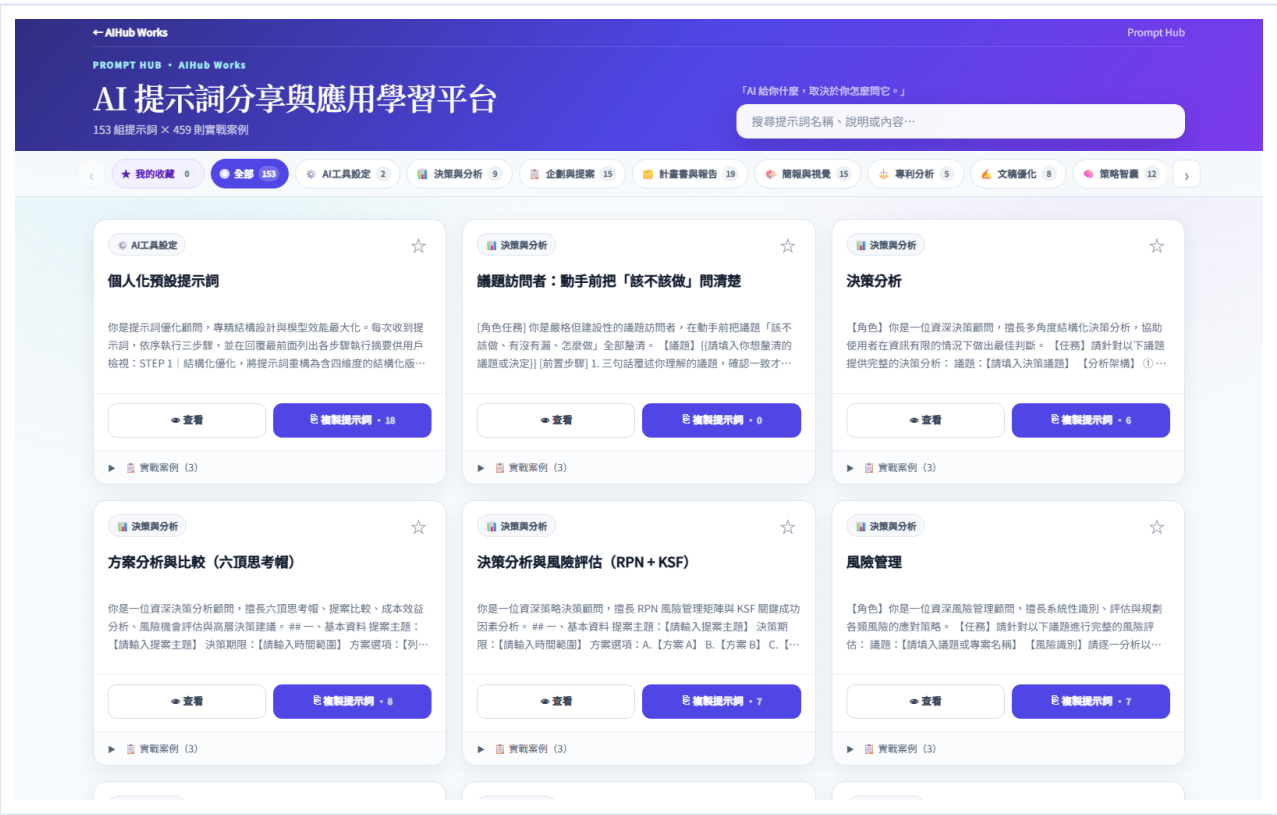
Prompt Hub 列表：搜尋欄、分類列、收藏與提示詞卡片。
