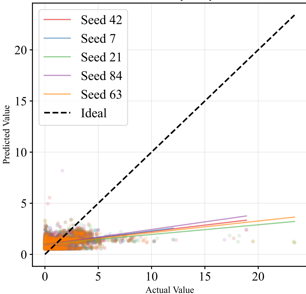
LASSO - Popularity
