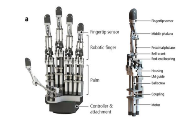
그림 2. 로봇 손 도식도
