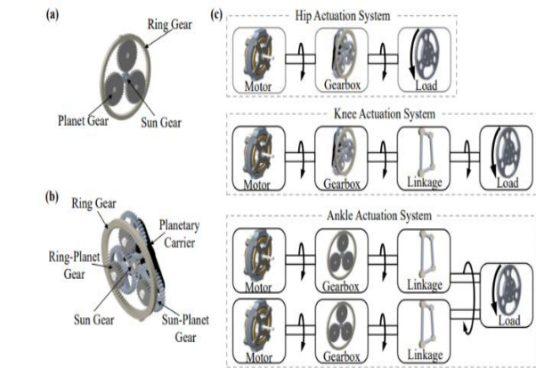
그림 1. 액추에이터 구성 부품
