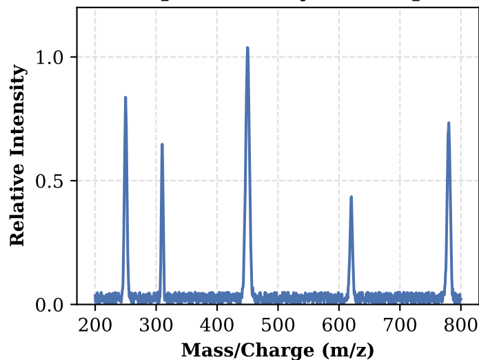
(d) Mass Spectrometry Data (Spectrum)
