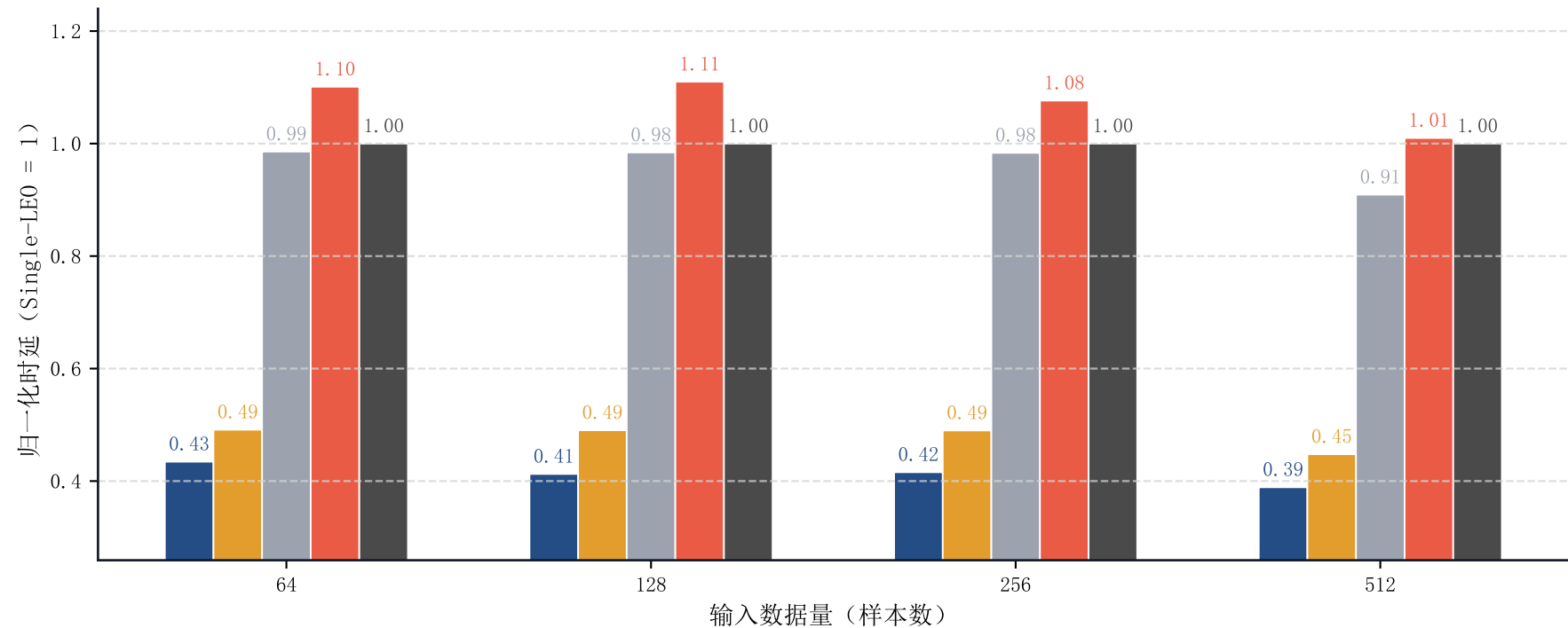
CDP模式下不同算法的归一化时延对比
