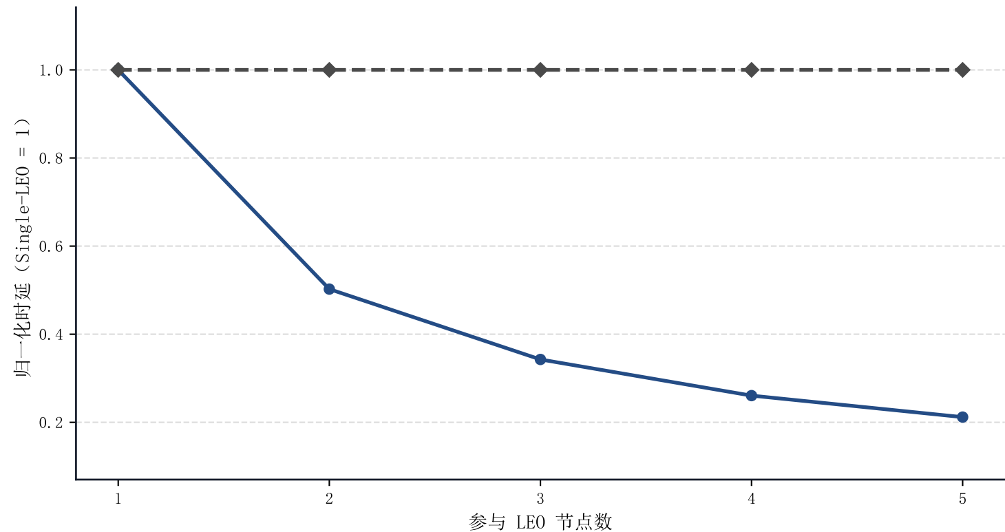
CDP 节点数与归一化时延
