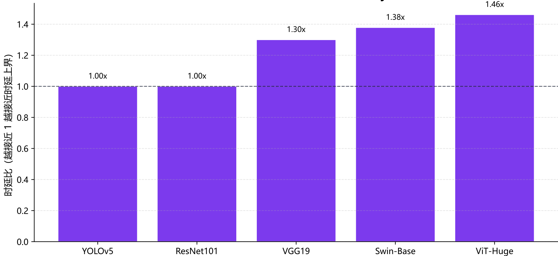
FWMS-Feature 相对 Oracle-Min-Latency 的时延比
