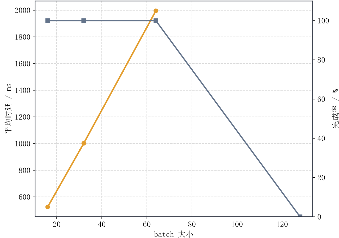
CDP 对 batch 的时延敏感性
