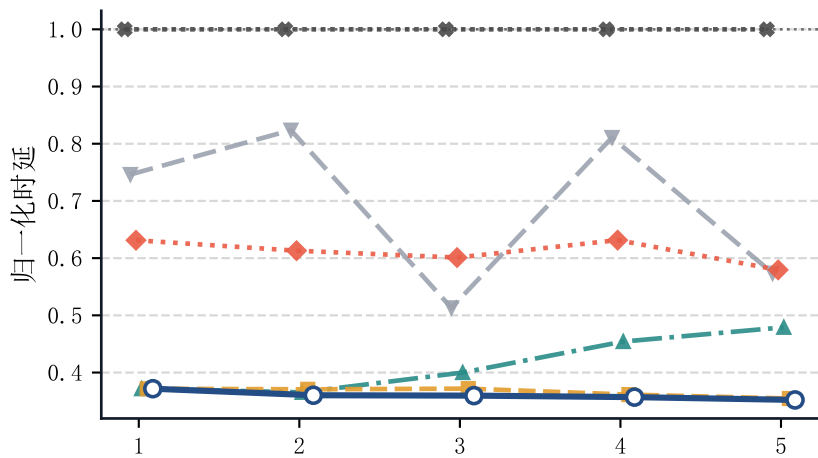
YOLOv5
