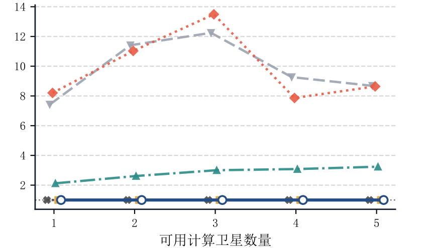
ViT-Huge
