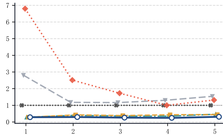
VGG19
