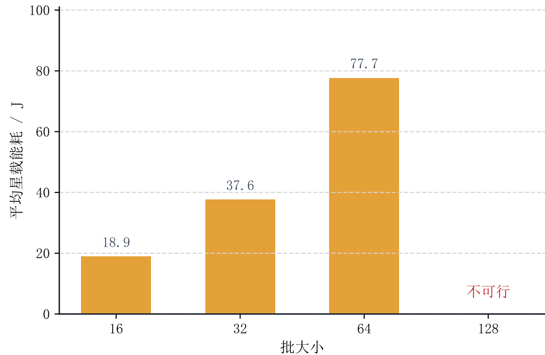
不同批大小下的 CDP 星载能耗
