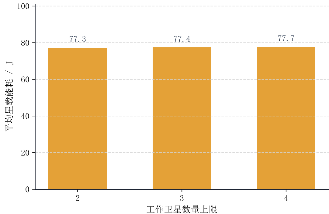
不同工作卫星数量下的 CDP 星载能耗
