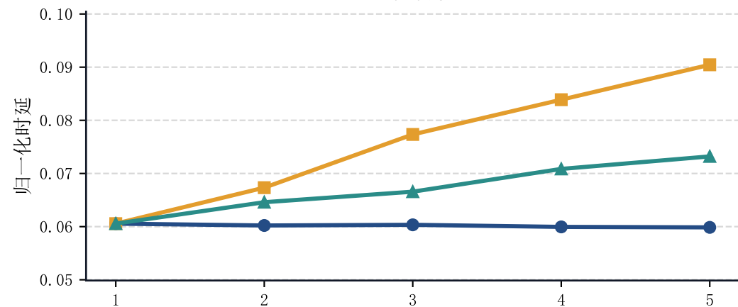
YOLOv5
