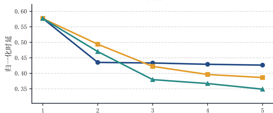
VGG19
