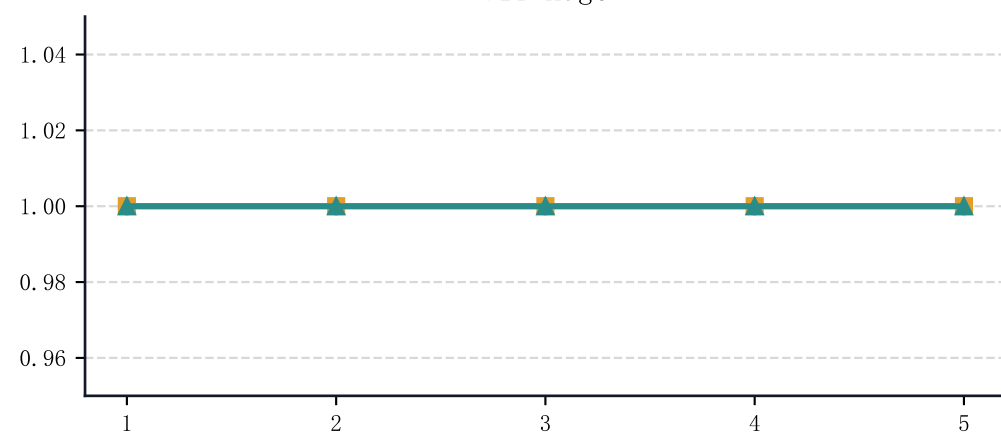
ViT-Huge
