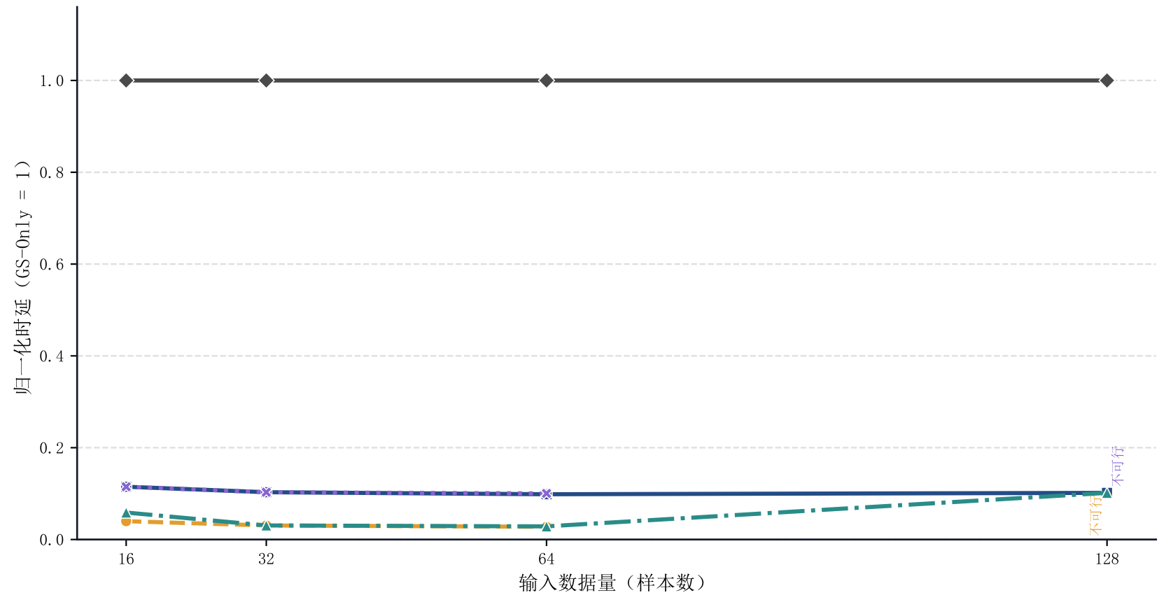
实验6：同时切片输入数据量敏感性（归一化，YOLOv5）
