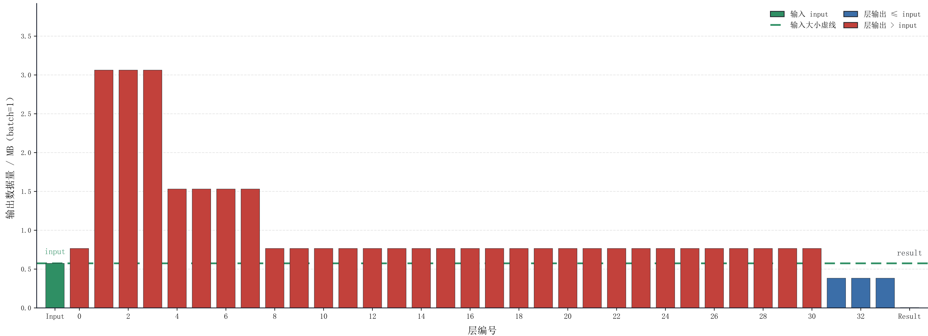
ResNet101 层级输出特征图数据量分布
