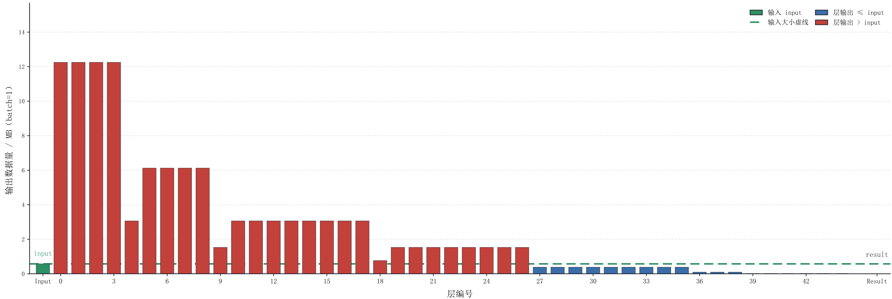
VGG19 层级输出特征图数据量分布
