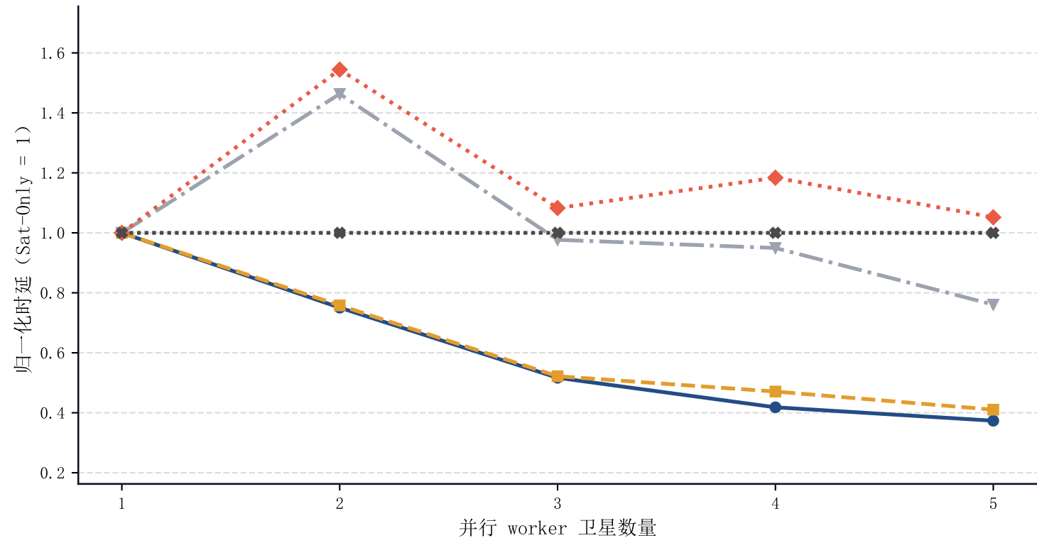
LAWA-CDP 模式的 worker 数量敏感性实验
