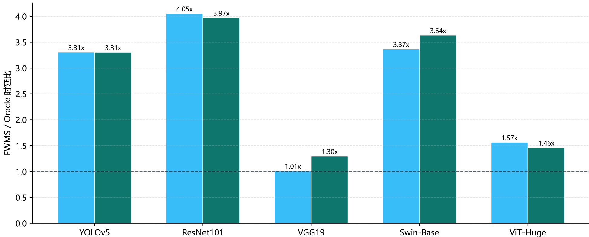
不同 batch 下 FWMS-Feature 相对 Oracle 的时延比
