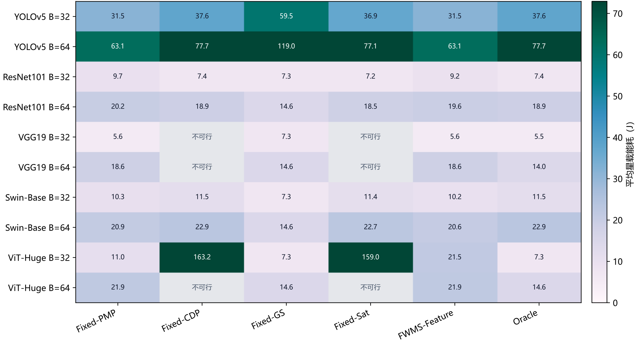
固定模式与 FWMS 的平均星载能耗对比
