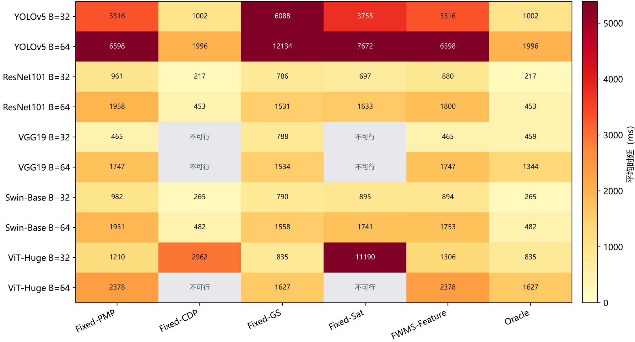
固定模式与 FWMS 的平均时延对比
