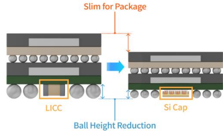
<그림6> LICC 대비 SiCap 적용 시 패키지 박형화 가능
