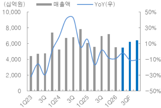
그림 1. 매출액 추정(YoY)
