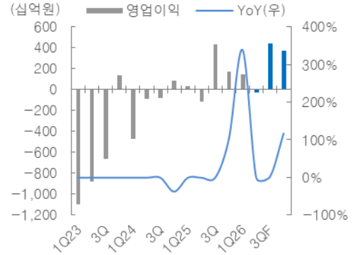
그림 2. 영업이익 추정(YoY)
