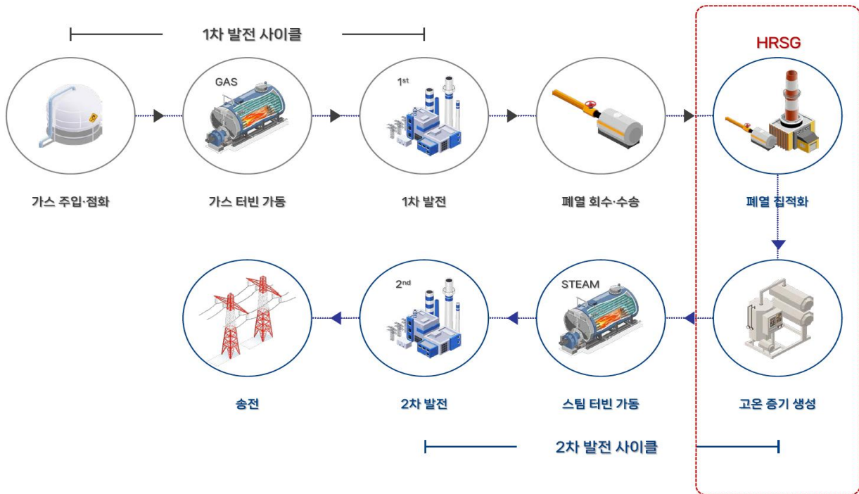
그림11. HRSG 기술개요
