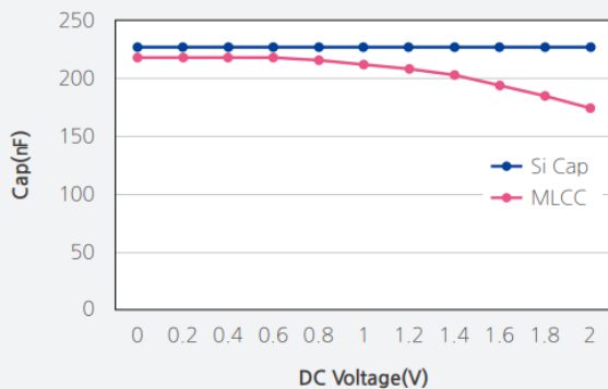
그림14 실리콘 캐패시터의 DC Bias 특성
