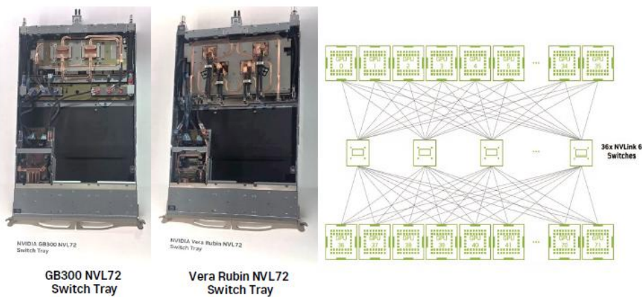
그림27 단일 랙 기준 NVSwitch 탑재량도 18개 → 36개로 증가
