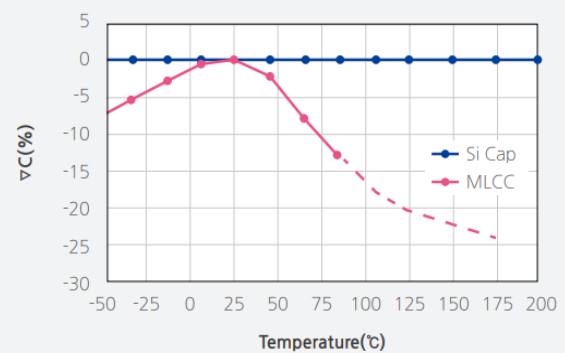
그림15 실리콘 캐패시터의 온도 안정성
