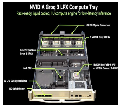
그림29 LPX = 32개의 LPU Tray = Tray당 8개의 LPU 사용
