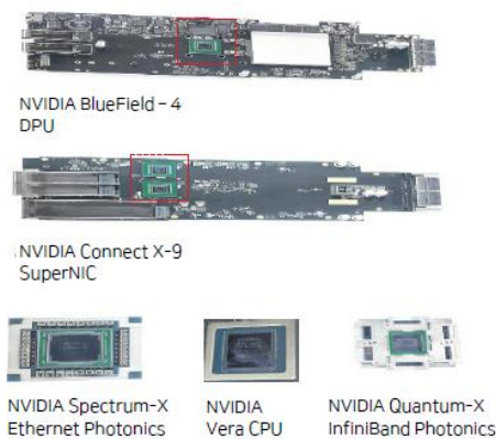
그림28 칩 기능의 세분화로 다양하게 사용되는 FC-BGA
