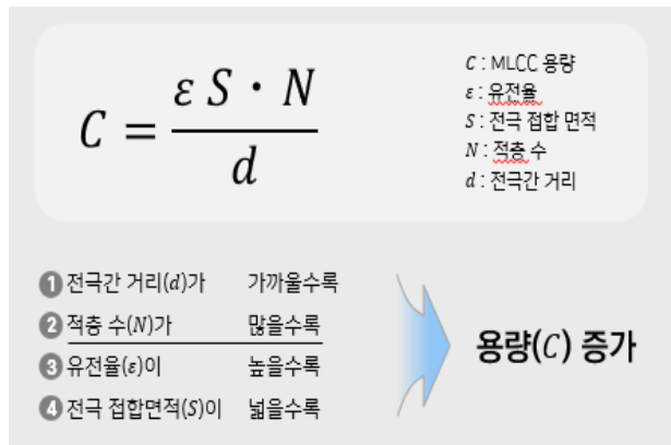
그림23 MLCC 용량 공식
