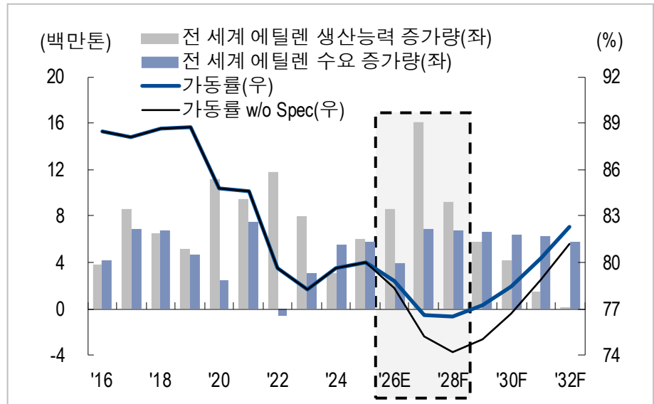
전 세계 에틸렌 가동률은 2028년까지 하락할 전망
