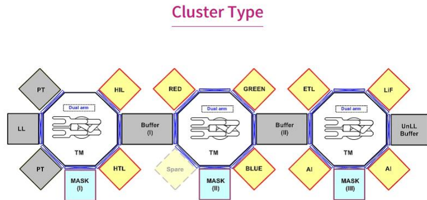
그림1. 선익시스템 증착장비의 핵심 기술 구조
