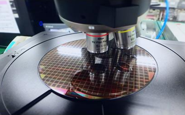
그림3 아이텍 PROVE TEST 공정과정
