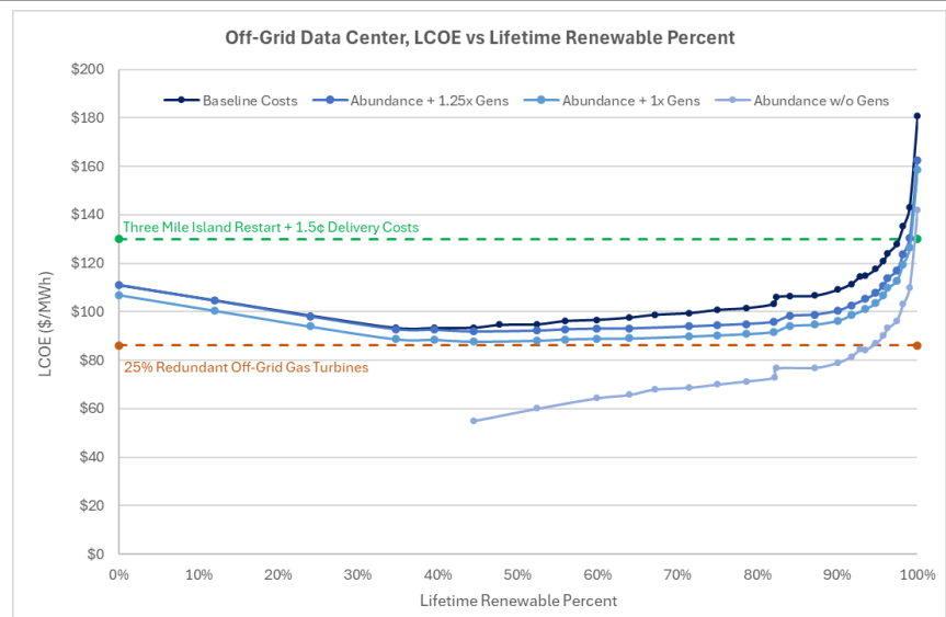
도표 88. 초기 태양광+ESS로 경제성 확보. 향후 발전기 Gas Generator 추가
