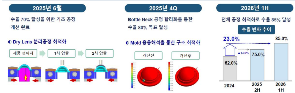
그림 8. 공정 수율 개선 노력
