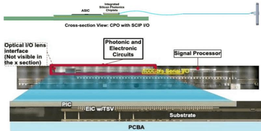
그림7. CPO의 단면도, ASIC 바로 옆에 광회로를 붙여 초고속, 저전력 통신을 구현
