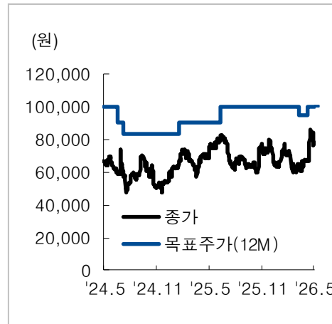
F&F (383220.KS)
