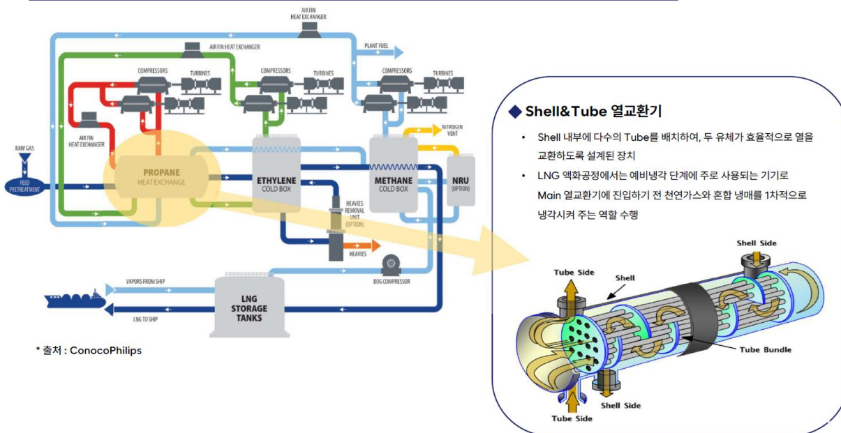
[도표 2] 한텍의 에너지사업부 핵심제품 Shell&amp;Tube 열교환기
